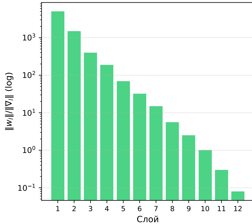
LARS: коэффициент масштабирования
