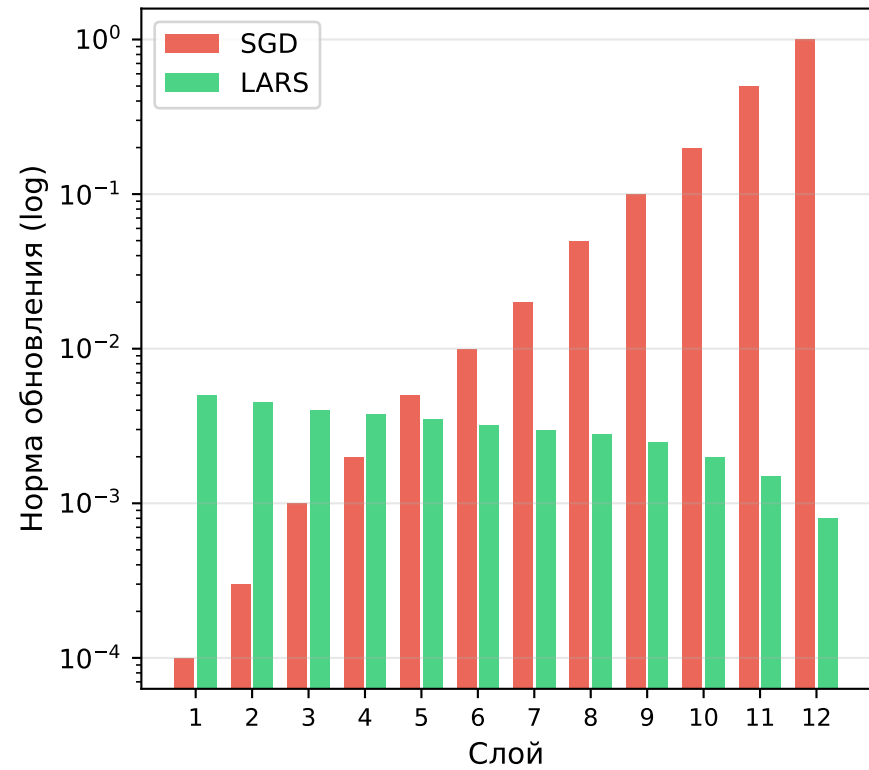
Эффективные обновления
