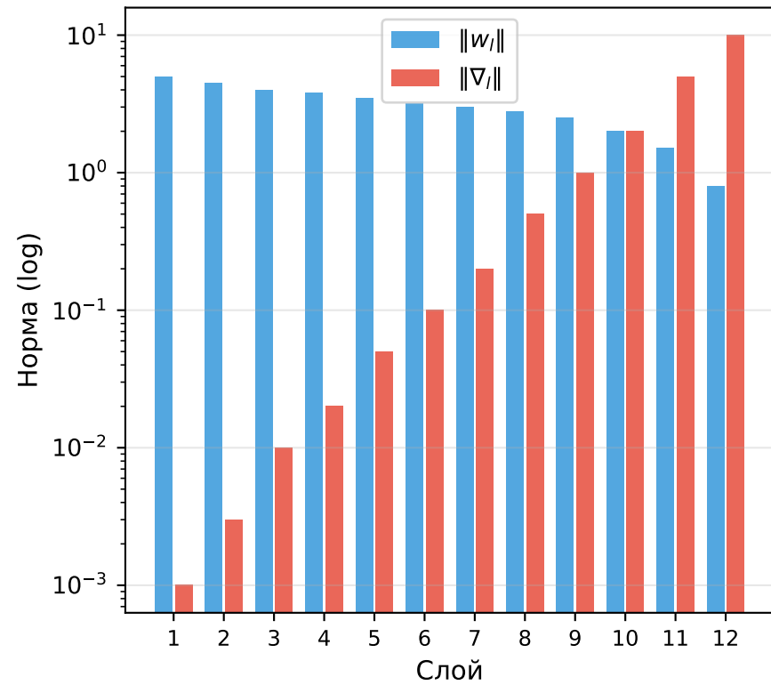
Нормы весов и градиентов
