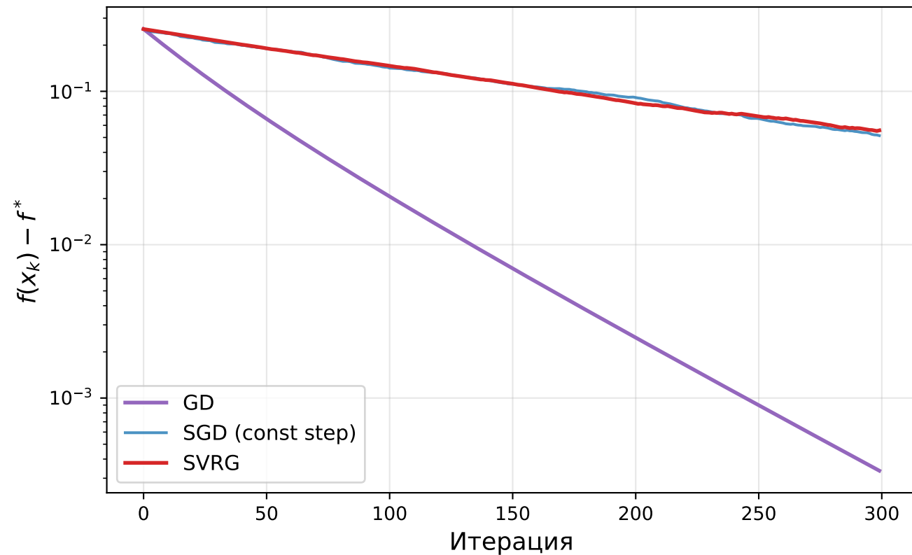
Сходимость
