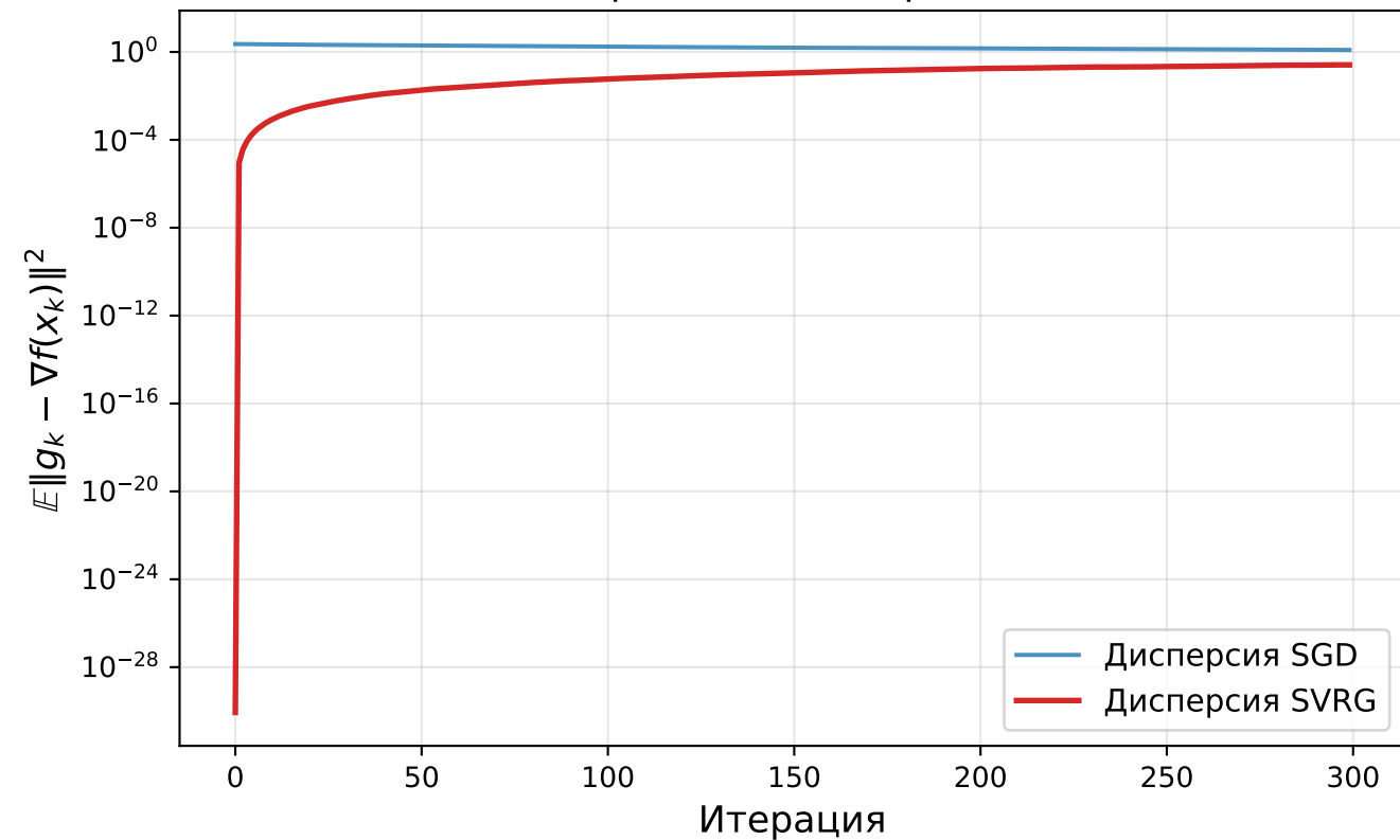
Дисперсия оценки градиента
