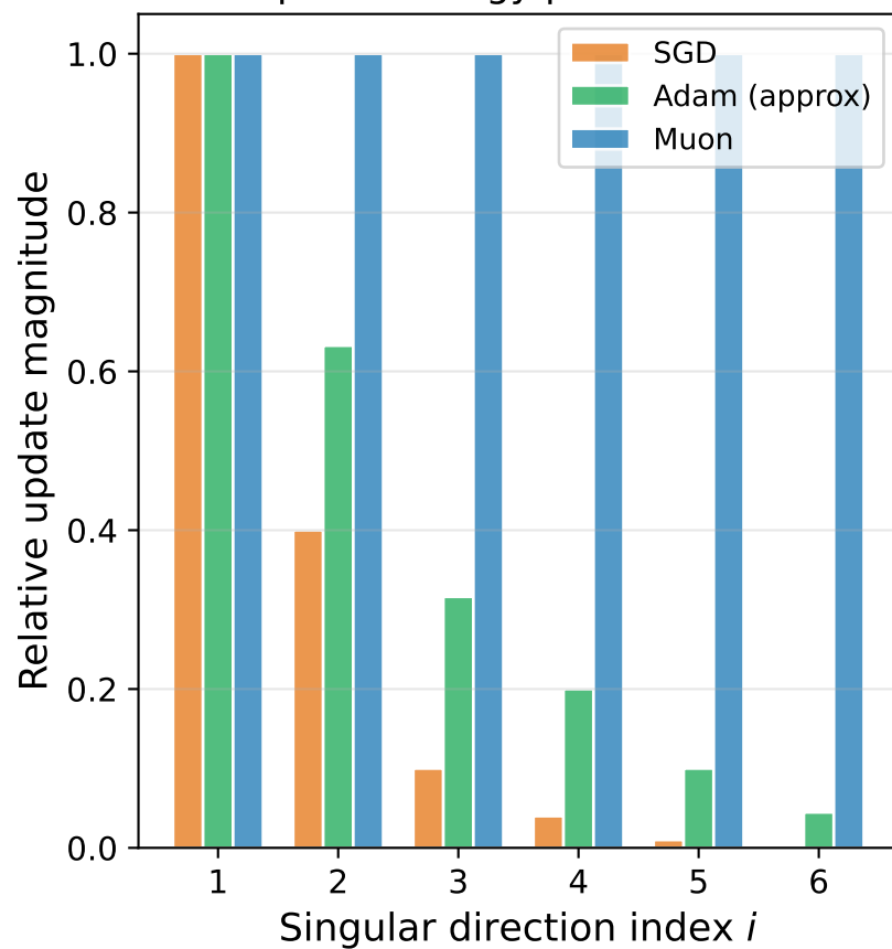
Update energy per direction
