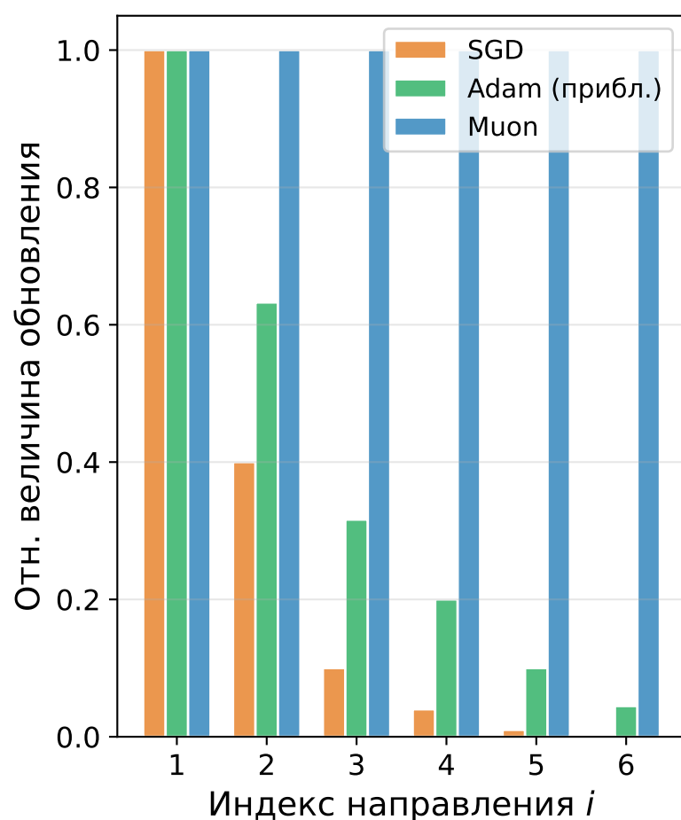
Энергия обновления по направлениям
