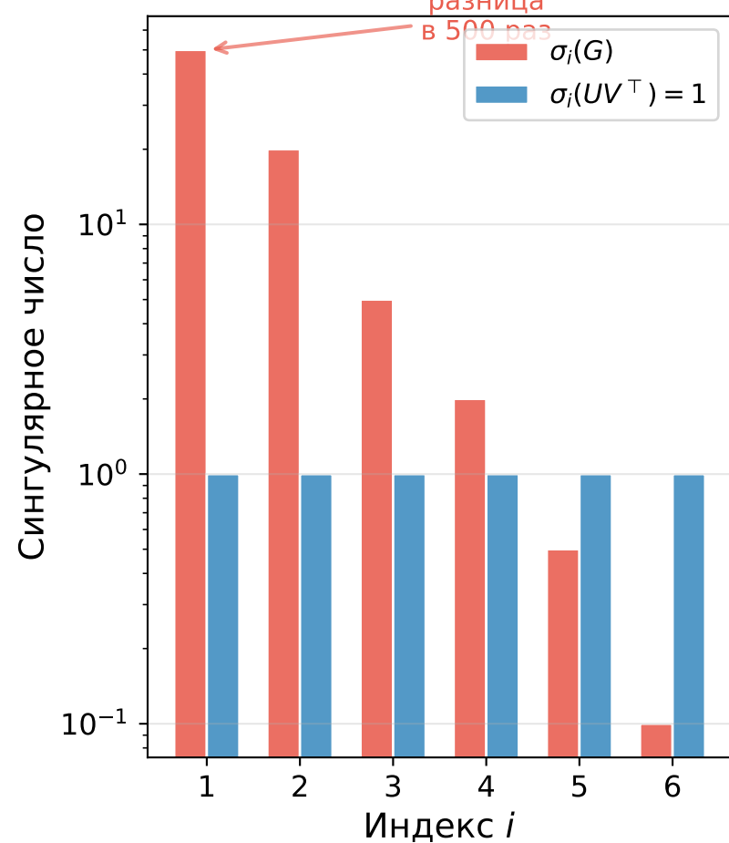
Сингулярные числа градиента и Muon
