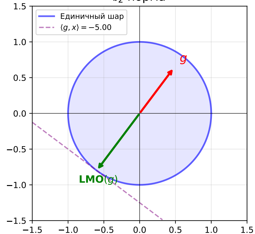
\ell_2 норма
