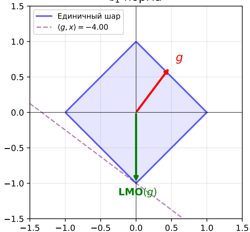
\ell_1 норма
