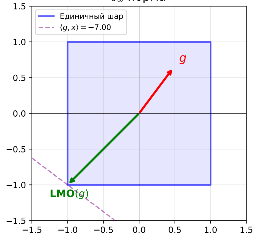
\ell_\infty норма
