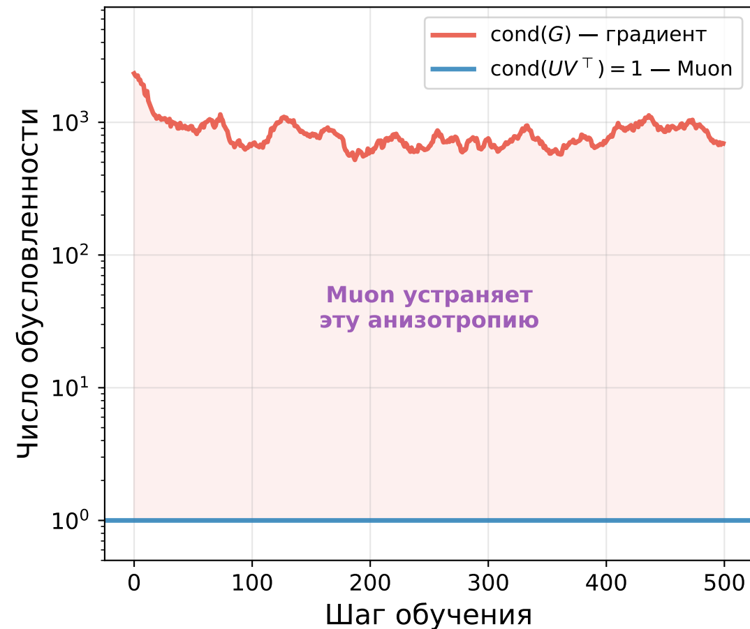
Число обусловленности
