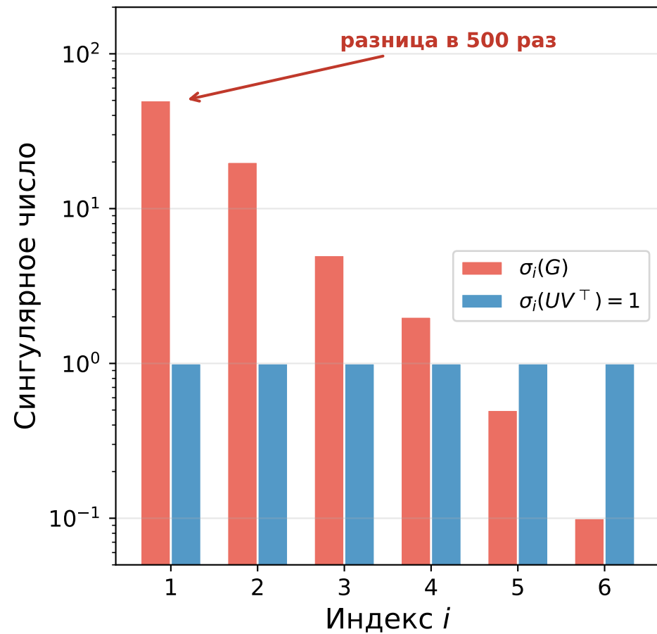
Сингулярные числа градиента и Muon
