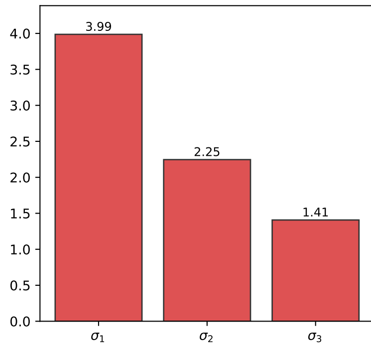
Синг. числа G
