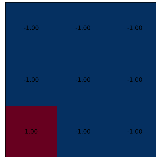
Синг. числа -\text{sign}(G)
