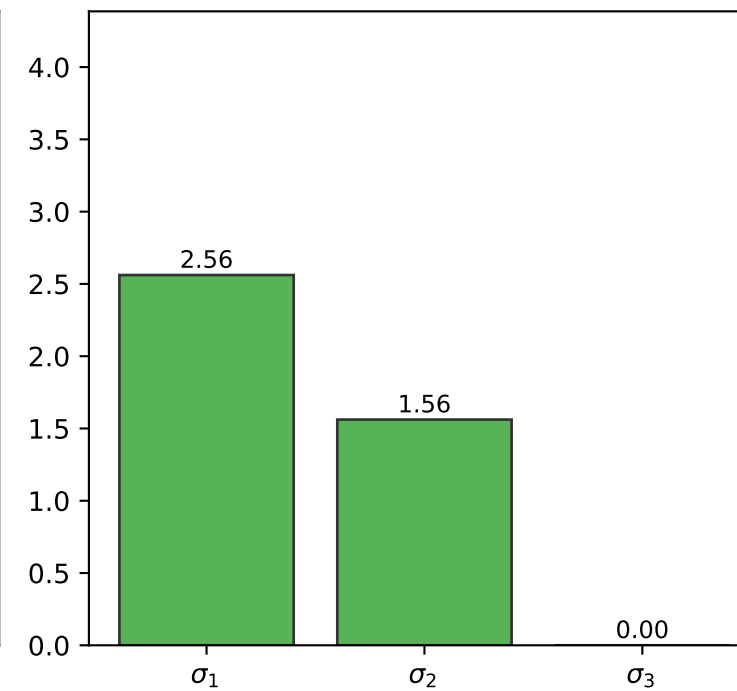
Синг. числа -\text{sign}(G)
