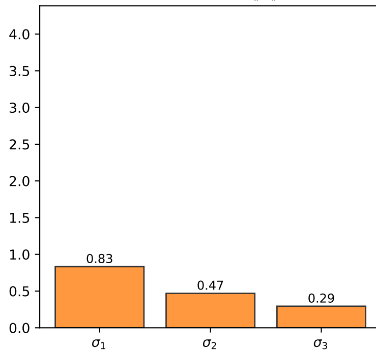
Синг. числа -G/\|G\|_F
