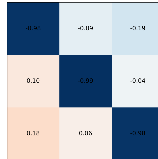
Синг. числа -UV^\top
