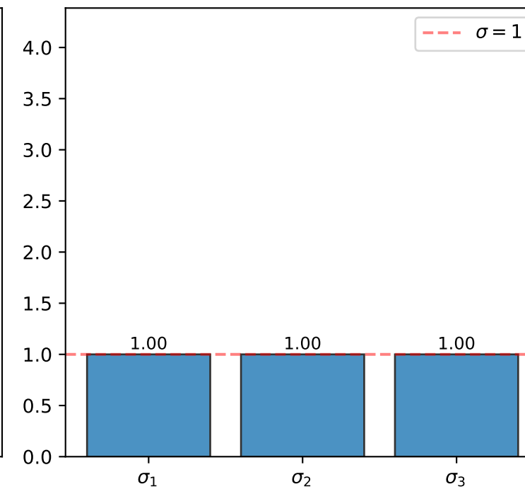
Синг. числа -UV^\top
