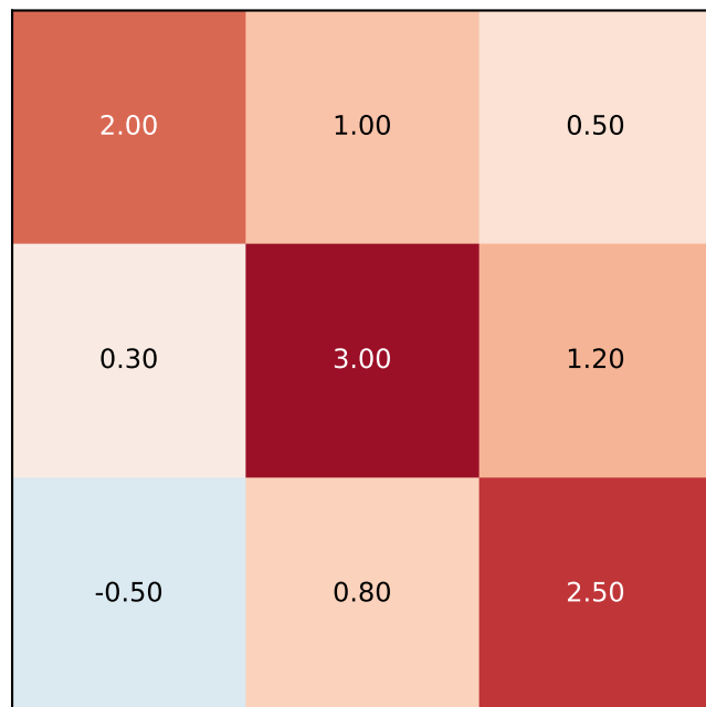
Синг. числа G
