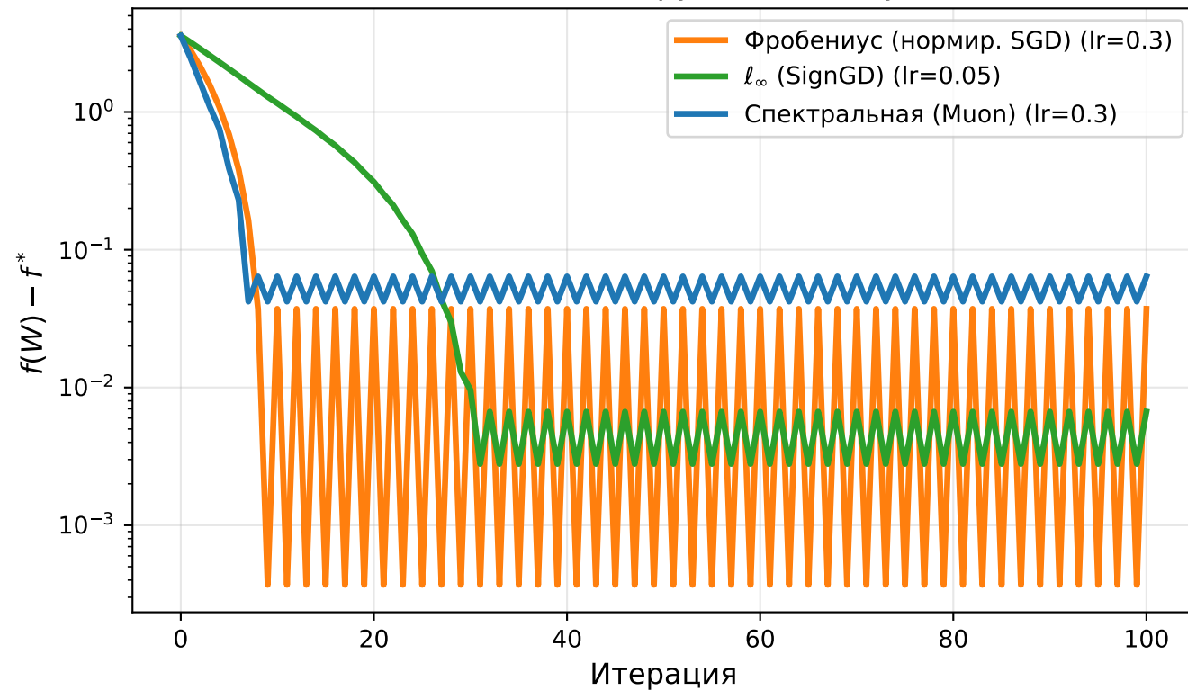
Сходимость наикрутейшего спуска
