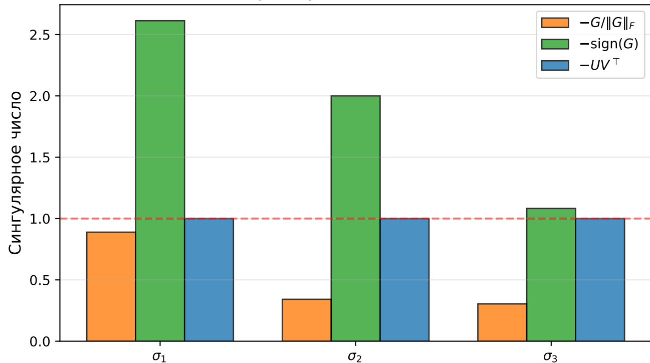
Спектр направления обновления
