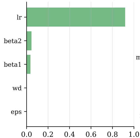
AdamW
