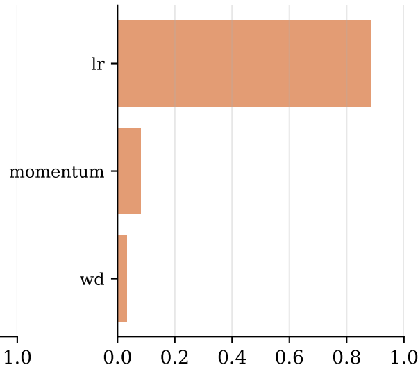
Nesterov
