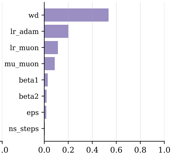
Muon
