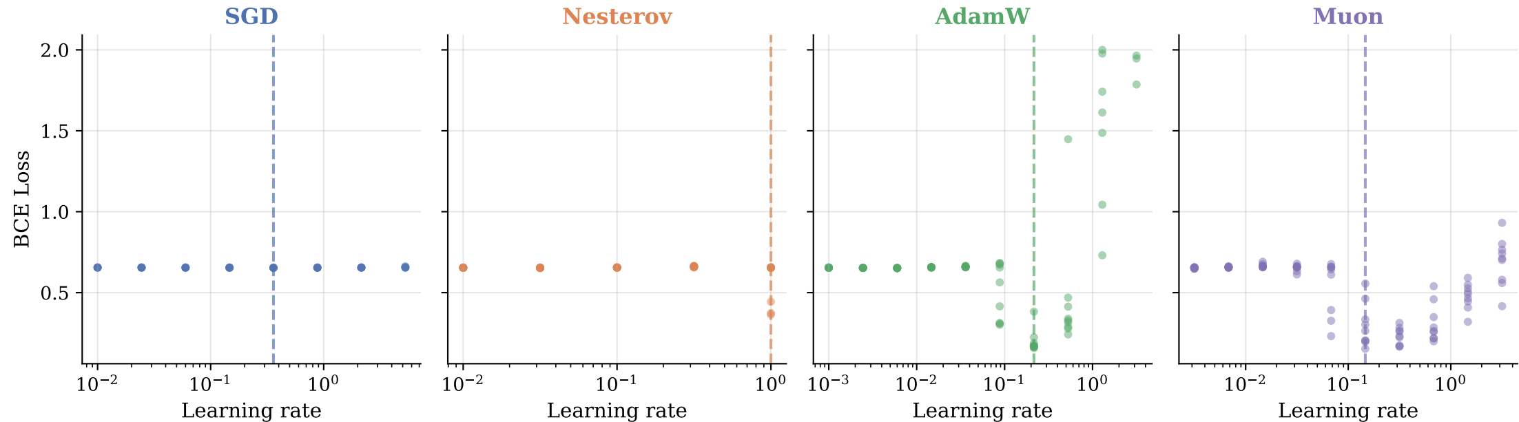
Чувствительность к learning rate (каждая точка = 1 конфигурация)
