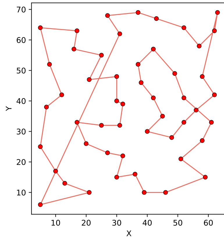
SA + 2-Opt Distance: 452.00
