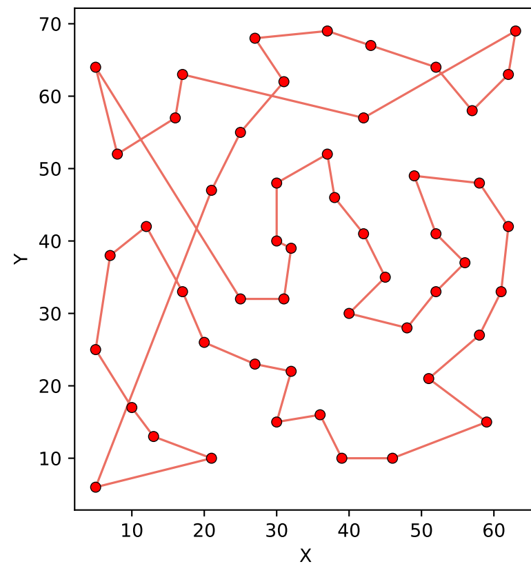
SA + 2-Opt Distance: 455.99
