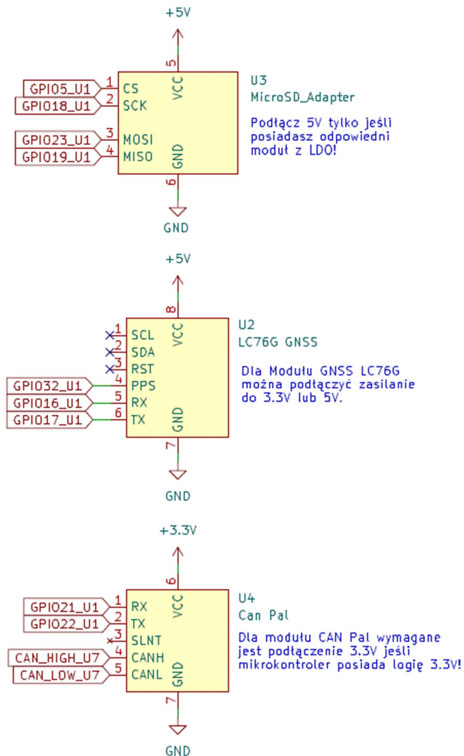
Rys. 4.10. Schemat połączeniowy peryferiów
