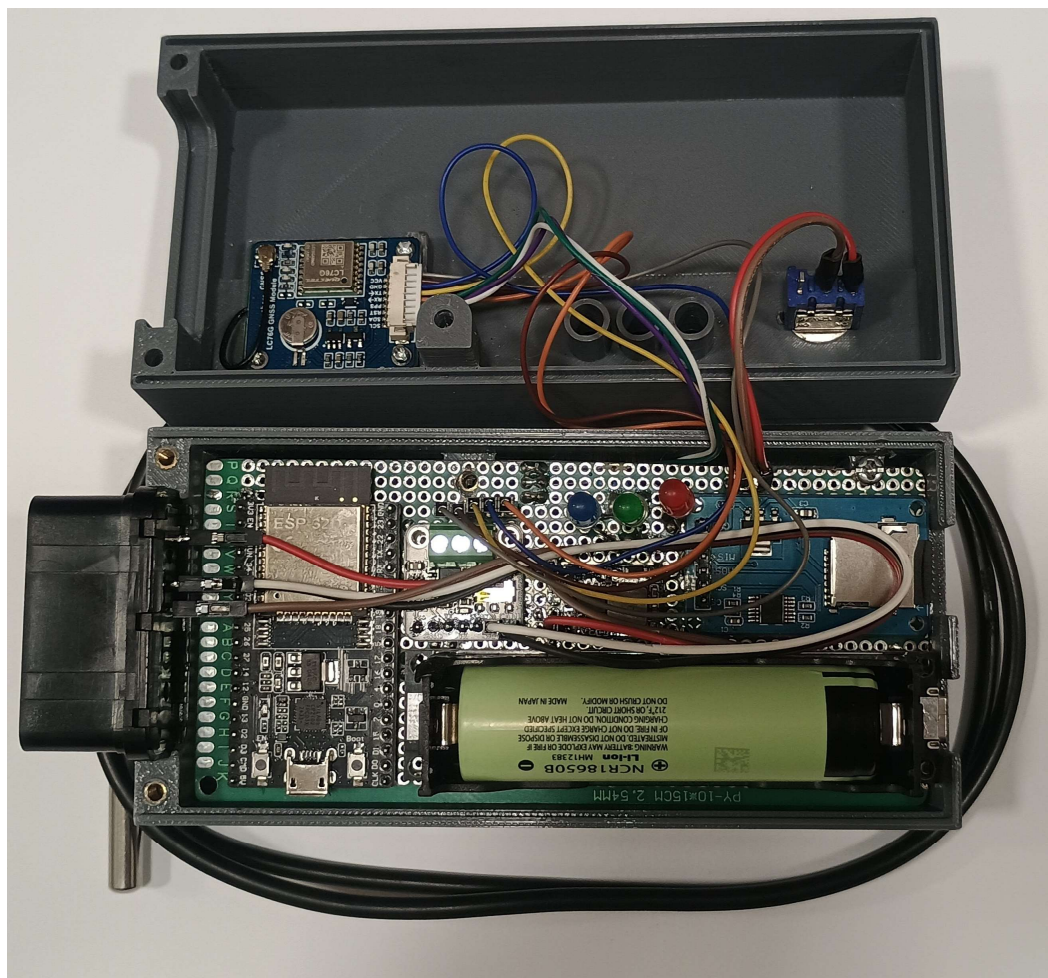
Rys. 4.11. Widok otwartego prototypu urządzenia. Widoczne osadzone ESP32 oraz moduły peryferyjne na płytce uniwersalnej.
