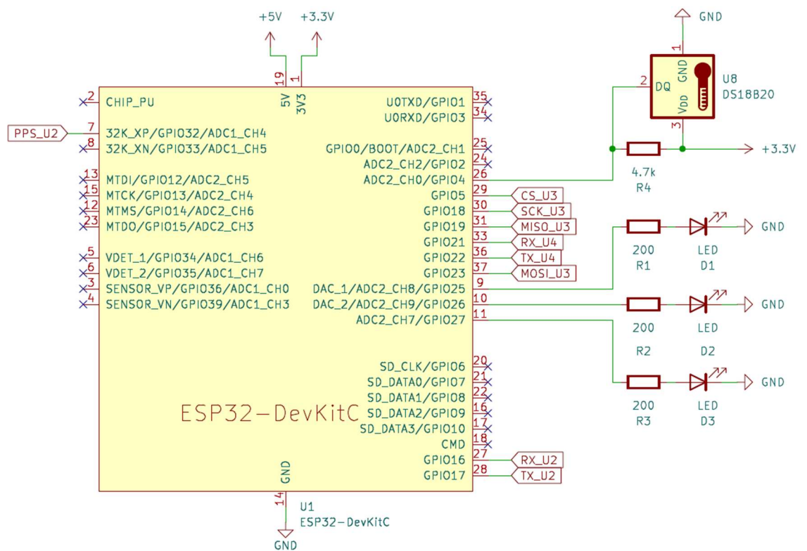
Rys. 4.8. Schemat połączeniowy ESP32
