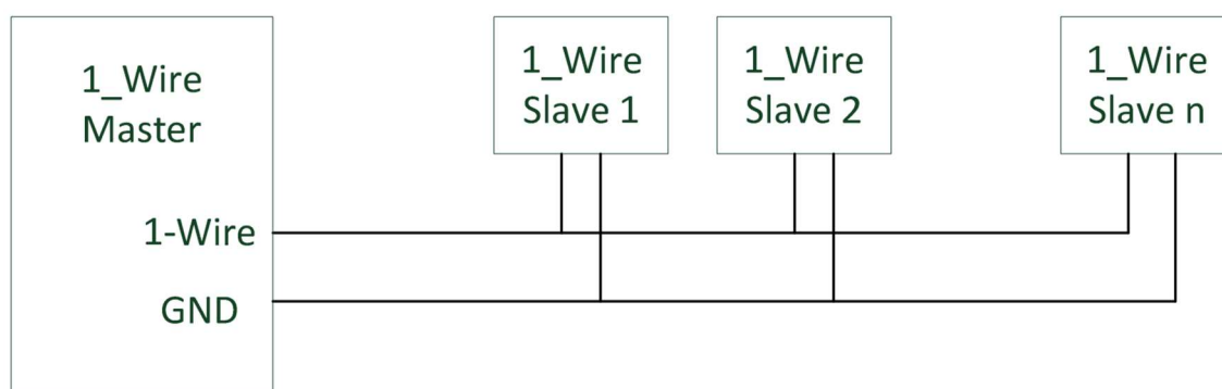
Rys. 3.3. Podstawowy schemat sieci 1-Wire. [5]
