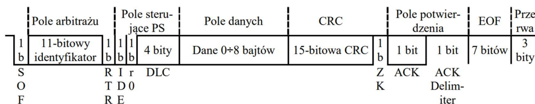
Rys. 3.1 Struktura ramki danych (format ramki standardowej – CAN 2.0A) [2]
