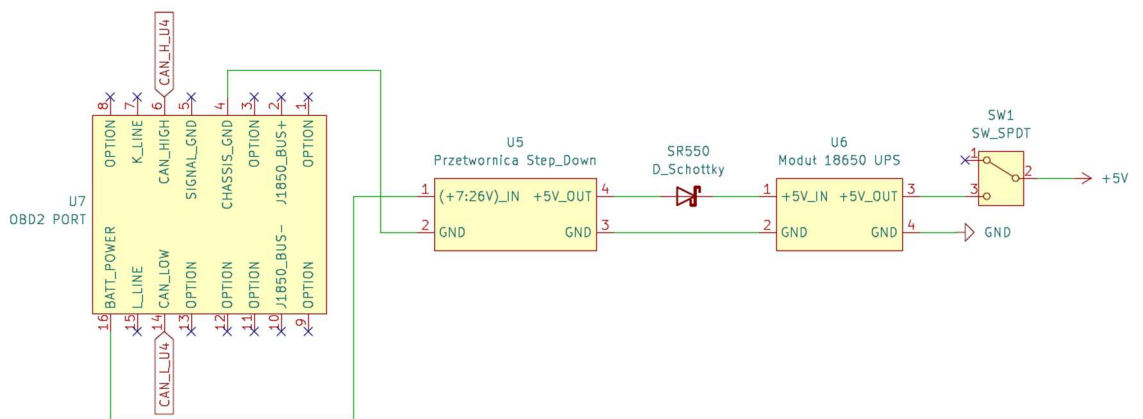
Rys. 4.9. Schemat połączeniowy zasilania
