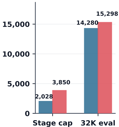
AIME24
