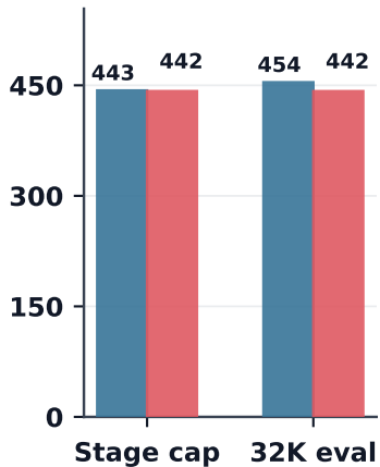
GSM8K
