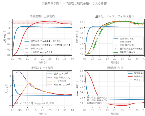
図 25: 実装条件による閉ループ応答、測定信号、実入力、状態制約余裕の変化。一次遅れ対象を同じ制御器で追従させ、理想的な離散実装と、 T_s = 0.08 [s]、計算遅れ T_c = 0.06 [s]、量子化幅 \Delta y = 0.025 、移動平均長 M = 5 、入力範囲 [-1.25, 1.25] 、レート制限 \Delta u_{max} = 0.18 /周期を含む実装を比較している。
