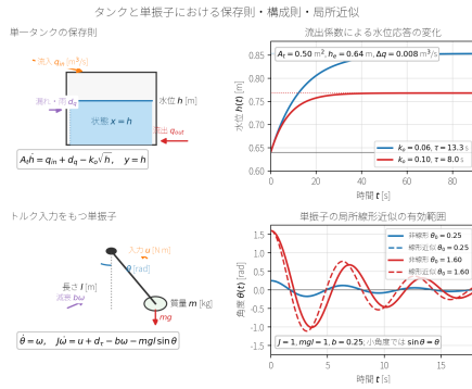
図 3: タンク水位モデルと単振子モデルの構造。タンクでは体積保存則と流出構成則から水位の状態方程式が得られ、流出係数 k_o を変えると線形化後の時定数と定常水位変化が同時に変わる。単振子ではトルク、重力、粘性減衰から角度と角速度の状態方程式が得られ、小角度では線形近似と非線形応答が一致しやすいが、大振幅では周期と振幅がずれる。
