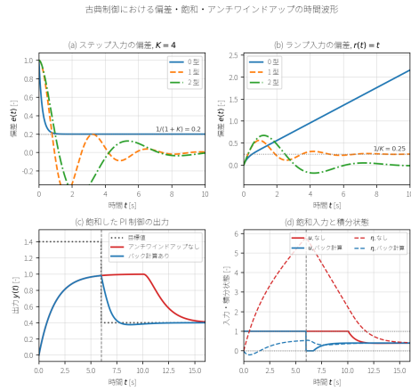
図 9: 系の型による定常偏差と、飽和時の PI 制御におけるアンチwindアップ効果。上段は L_0(s) = 4/(s+1) , L_1(s) = 4/\{s(s+1)\} , L_2(s) = 4(s+1)/\{s^2(s+4)\} の単位負帰還を同じ入力で比較し、型が上がると追従できる基準入力の次数が一つずつ上がることを示す。下段は P(s) = 1/(1.5s+1) , K_P = 2.0 , K_I = 1.5 , 0 \leq u \leq 1 の PI 制御で、バック計算が飽和中の積分状態を入力制約に合わせて戻すことを示す。
