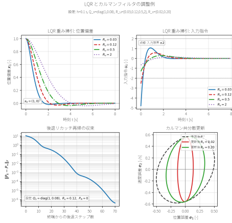
図 15: 二重積分器に対する LQR と Kalman フィルタの調整例。上段は入力重み R_u による状態応答と入力指令の変化であり、入力限界を点線で示している。左下は有限ホライズンの後退リカッチ再帰が定常解へ近づく様子である。右下は予測後の誤差共分散楕円が位置測定によって更新される様子であり、測定ノイズ分散 R_v が小さいほど測定方向の不確かさが強く縮む。
