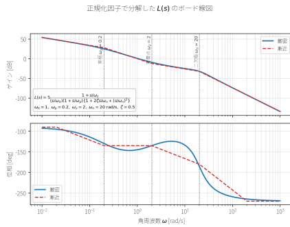
図 7: 正規化された開ループ L(s) のボード線図。0.2 rad/s の実極でゲイン傾きが下がり、2 rad/s の実零点で戻り、20 rad/s の二次極でさらに低下する。破線の漸近線と実線の厳密線図を比べると、折点近傍の誤差と位相遷移を確認できる。
