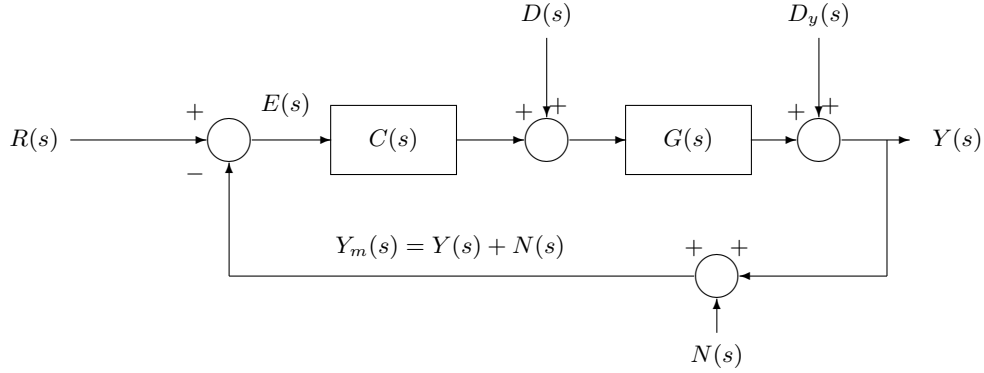
図 5: 目標値、制御器、対象、外乱、測定ノイズを含む負帰還ブロック線図
