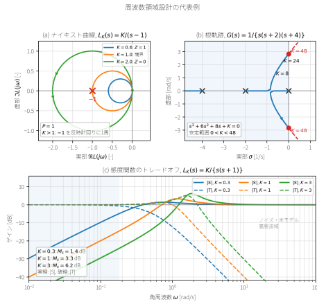
図 8: ナイキスト線図、根軌跡、感度関数を同じ周波数設計の確認図として並べた例。上左は不安定開ループ極 P = 1 を持つ L_K(s) = K/(s-1) のゲイン変化で、 K > 1 だけが点 -1 を反時計回りに 1 回囲み閉ループが安定になる。上右は三次開ループ G(s) = 1/\{s(s+2)(s+4)\} の根軌跡で、 0 < K < 48 が安定範囲、 K = 48 で虚軸を横切る。下は L_K(s) = K/\{s(s+1)\} の S と T で、ゲインを上げるほど低周波の外乱抑制は強くなるが、感度ピークと相補感度の通過帯域が増える。
