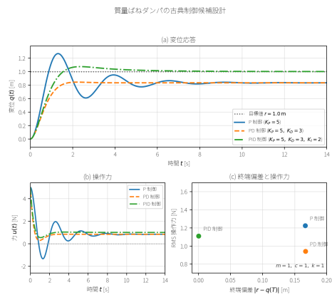
図 10: 質量ばねダンパ系に対する P、PD、PID 候補設計の比較。対象は m = 1 \text{ kg} 、 c = 1 \text{ N s/m} 、 k = 1 \text{ N/m} 、目標値は r = 1 \text{ m} である。PD 制御は速度フィードバックで振動を抑え、PID 制御は積分状態で定常偏差を減らす、操作力の使い方も変わる。
