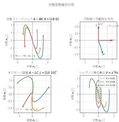
図 14: 二状態モデル A = \begin{bmatrix} 0 & 1 \\ -2 & -3 \end{bmatrix} , b = \begin{bmatrix} 0 & 1 \end{bmatrix}^T , C = \begin{bmatrix} 1 & 0 \end{bmatrix} に対する状態空間の幾何。左上は K = \begin{bmatrix} 18 & 6 \end{bmatrix} による閉ループ軌道、右上は可制御方向 B, AB と可観測方向 C^T, A^T C^T 、左下は L = \begin{bmatrix} 10 & 10 \end{bmatrix}^T による推定誤差軌道、右下は A - bK に対する V = x^T P x のレベル集合を示す。
