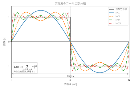
図 6: 周期 2\pi 、振幅 \pm 1 に正規化した方形波と、奇数次高調波 k = 1, 3, \dots, N だけを N = 1, 3, 9, 25 で打ち切ったフーリエ部分和。高い奇数次高調波ほど不連続点近傍の鋭い立上りを作るため、帯域制限をもつ制御対象や閉ループでは方形波指令や急な外乱が丸められ、帯域付近の位相遅れや共振が過渡応答として現れやすい。
