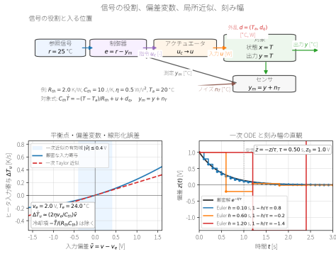
図 1: 信号の役割、偏差変数、局所線形化、数値積分刻み幅の対応。上段は熱系における参照信号、入力、出力、外乱、ノイズ、状態の入る位置を示す。左下は T_a = 20^\circ\text{C} 、 R_{\text{th}} = 2.0 \text{ K/W} 、 C_{\text{th}} = 10 \text{ J/K} 、 \eta = 0.5 \text{ W/V}^2 、 v_e = 2.0 \text{ V} の動作点で、ヒータ電圧偏差 \tilde{v} が温度変化率へ与える入力寄与 \Delta \dot{T}_u とその一次 Taylor 近似を比較している。完全な線形化式には、これに加えて冷却による -\tilde{T}/(R_{\text{th}}C_{\text{th}}) も入る。右下は \dot{z} = -z/\tau 、 \tau = 0.50 \text{ s} に陽的 Euler 法を適用し、刻み幅 h によって精度と数値安定性が変わることを示す。
