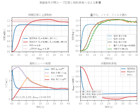
図 21: 実装条件による閉ループ応答、測定信号、実入力、状態制約余裕の変化。一次遅れ対象を同じ制御器で追従させ、理想的な離散実装と、 T_s = 0.08 [s]、計算遅れ T_c = 0.06 [s]、量子化幅 \Delta y = 0.025 、移動平均長 M = 5 、入力範囲 [-1.25, 1.25] 、レート制限 \Delta u_{\max} = 0.18 /周期を含む実装を比較している。
