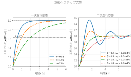
図 4: 正規化した一次遅れ応答と二次遅れ応答の比較。左は y/(Ku_0) = 1 - e^{-t/\tau} において時定数 \tau だけを変えたステップ応答であり、各曲線は t = \tau で 1 - e^{-1} に達する。右は \omega_n = 2 \text{ rad/s} を固定し、減衰比 \zeta を変えた標準二次系の単位ステップ応答である。
