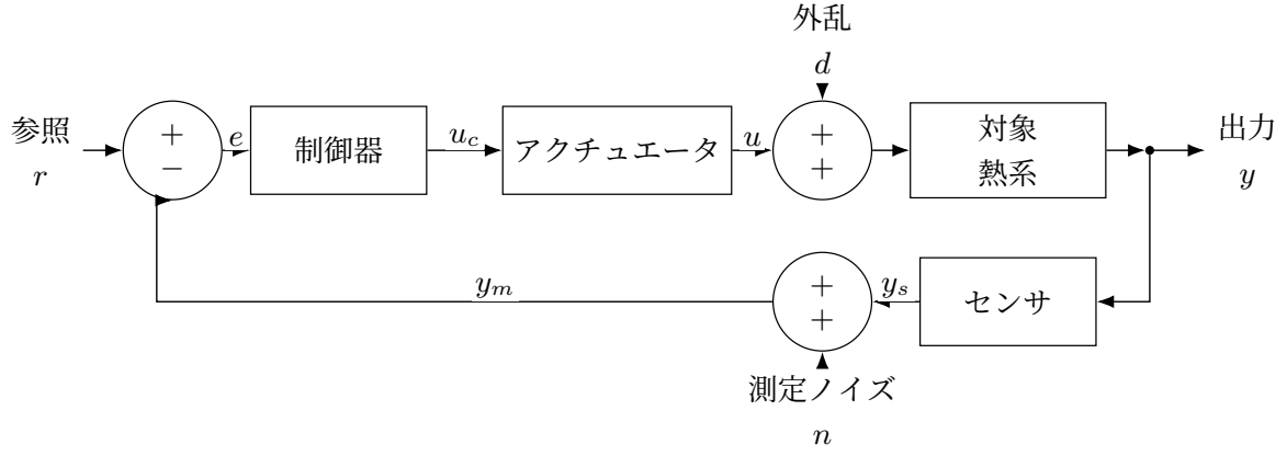
図 2: 熱系における参照信号、制御器、アクチュエータ、対象、センサ、外乱、ノイズの入る位置。外乱は対象の状態を変え、ノイズはセンサ測定値に加わる。
