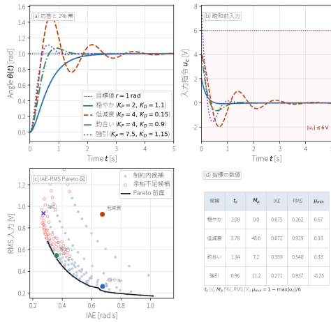
図 22: DC モータ位置サーボに対する性能指標と Pareto 図。対象は J = 0.20 \text{ kg m}^2 、 b = 0.25 \text{ N m s/rad} 、 K_t = 1.0 \text{ N m/V} 、入力制約は |u| \leq 6.0 \text{ V} 、目標値は r = 1.0 \text{ rad} である。上段は応答と飽和前入力、下段左は多数の K_P, K_D 候補を IAE と RMS 入力で比べた Pareto 図、下段右は代表候補の指標表である。
