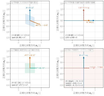
図 29: 可制御性、可観測性、PBH 条件の幾何的な比較。左上は A = \begin{bmatrix} 0 & 1 \\ -2 & -0.4 \end{bmatrix} 、 B = \begin{bmatrix} 0 \\ 1 \end{bmatrix} としたとき、 B と AB が二次元平面を張り \text{rank } C = 2 となる例を示す。右上は B と AB が同一直線上に残り、 x_2 方向が到達不能になるため \text{rank } C = 1 へ落ちる例である。左下は C = [1 \ 0] としたとき、 C^T と A^T C^T が二次元平面を張り \text{rank } O = 2 となる例を示す。右下は A = \text{diag}(1, -2) 、 B = C^T = e_2 としたとき、不安定固有方向 e_1 が入力方向にも測定方向にも含まれず、 \lambda = 1 の PBH 行列ランクが 1 < 2 へ低下する例である。
