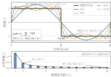
図 24: 周期 2\pi 、振幅 \pm 1 に正規化した方形波と、奇数次高調波 k = 1, 3, \dots, N だけを N = 1, 3, 9, 25 で打ち切ったフーリエ部分和。高い奇数次高調波ほど不連続点近傍の鋭い立上りを作るため、帯域制限をもつ制御対象や閉ループでは方形波指令や急な外乱が丸められ、帯域付近の位相遅れや共振が過渡応答として現れやすい。
