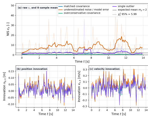
図 36: 二重積分器で近似した台車の位置・速度測定に対する革新 \nu_k と正規化革新二乗 \epsilon_k の例。上段では細線が各サンプルの \epsilon_k 、太線が 8 サンプル平均を表し、期待平均 m_y = 2 と \chi^2_2 の 95% 線を併記している。下段の革新成分を見ると、単発外れ値は孤立した大きな \nu_k と \epsilon_k のスパイクとして現れ、共分散全体をただちに更新すべき継続的な不整合とは区別できる。
