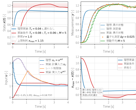
図 53: 実装条件による閉ループ応答、測定信号、実入力、状態制約余裕の変化。一次遅れ対象を同じ制御器で追従させ、理想的な離散実装と、 T_s = 0.08 [s]、計算遅れ T_c = 0.06 [s]、量子化幅 \Delta y = 0.025 、移動平均長 M = 5 、入力範囲 [-1.25, 1.25] 、レート制限 \Delta u_{\max} = 0.18 /周期を含む実装を比較している。
