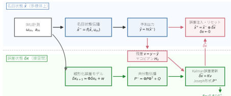
図 43: ESKF における名目状態と誤差状態の分離。IMU 測定は名目状態を伝搬し、同時に接空間上の誤差共分散を伝搬する。測定革新は誤差状態を更新し、推定された誤差は名目状態へ注入されてからリセットされる。
