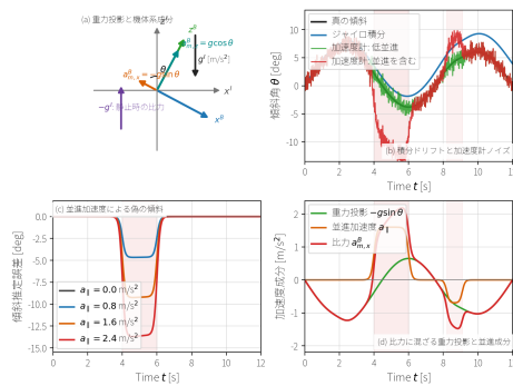
図 40: 加速度計による重力投影と傾斜推定の限界。左上は、静止時の比力が機体系の x^B, z^B 軸へ投影され、 a_{m,x}^B = -g \sin \theta 、 a_{m,z}^B = g \cos \theta になる幾何である。右上は、真の傾斜、ジャイロ積分、低並進時の加速度計傾斜、並進加速度を含む加速度計傾斜を比較している。左下は a_{||} = 0.0, 0.8, 1.6, 2.4 \text{ m/s}^2 の変化による偽の傾斜誤差、右下は比力の x 軸成分が重力投影と並進加速度の和として現れることを示す。
