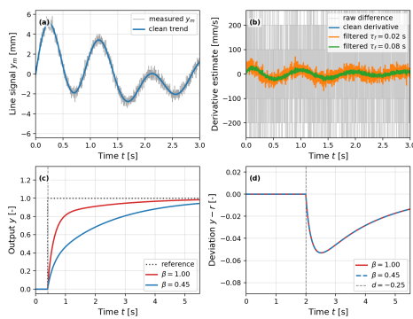
図 14: 微分フィルタと二自由度 PID の時間応答比較。上段はノイズを含むラインセンサ測定値 y_m [mm] と、その差分微分およびフィルタ付き微分を示す。 \tau_f を大きくするとノイズは減るが、真の変化への追従は遅れる。下段は P(s) = 1/(0.6s + 1) 、 K_P = 3.0 、 K_I = 1.8 、 K_D = 0.12 、 \tau_f = 0.04 s、 \gamma = 0 の二自由度 PID で、 \beta を下げると指令応答が穏やかになり、目標値を固定した外乱応答はほぼ変わらないことを示す。
