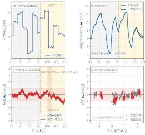
図 21: DC モータ速度応答の一次モデル同定と検証残差。上段左は入力電圧の時系列で、灰色を同定用データ、淡い黄色を検証用データとした。上段右は同定用データから得た \hat{K} = 7.78 \text{ rad/s/V} 、 \hat{\tau} = 0.43 \text{ s} の一次モデルを全区間へ適用した結果である。下段左は測定速度とモデル予測の差であり、検証区間の RMS 残差は 0.58 \text{ rad/s} 、最大絶対残差は 1.56 \text{ rad/s} である。下段右は入力電圧と残差の関係を表し、残差が入力や検証区間に依存している部分が未モデル化要素を表す。
