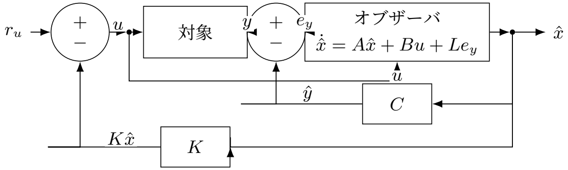
図 31: 推定状態を用いる状態フィードバックと Luenberger オブザーバの信号経路。対象とオブザーバには同じ制御入力 u が入り、測定値 y と推定出力 \hat{y} = C\hat{x} の差 e_y が推定誤差を修正する。
