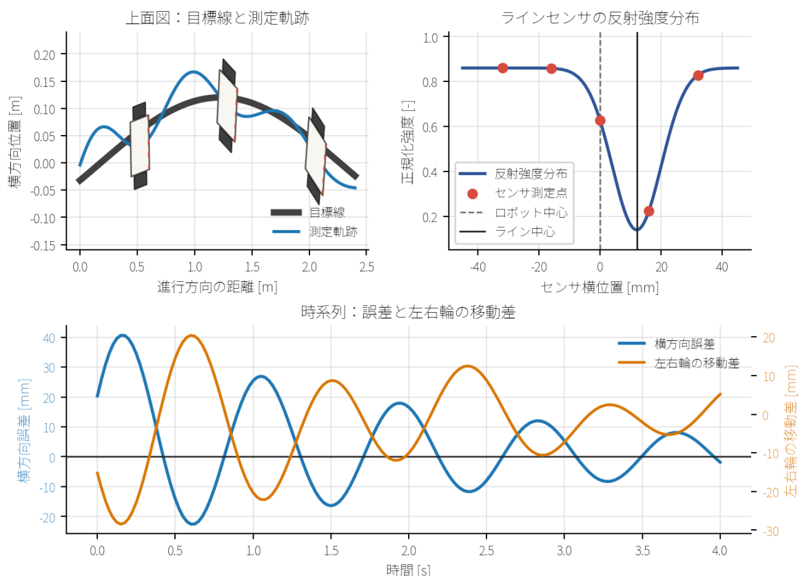
図 1: ライントレースロボットの観察から得られる最初の測定例。左上は床上の目標線と測定された走行軌跡のずれ、右上は横一列のラインセンサが線中心の偏りを強度分布として読む様子、下段は横方向誤差と左右輪の移動差の時間履歴を示す。
