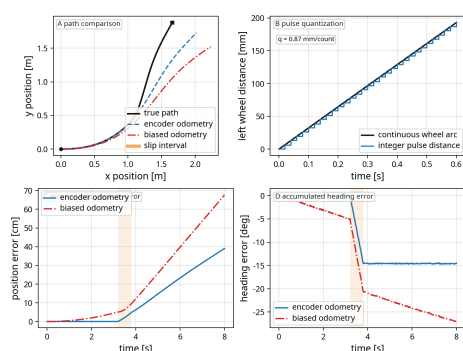
図 38: 差動二輪ロボットにおける真の経路、通常のエンコーダオドメトリ、半径誤差を重ねたオドメトリの比較。左車輪は 3.20–3.80 s だけすべり、車輪外周の移動量 0.204 m のうち 0.081 m が地面上の移動に変換されない。量子化の 1 count は 0.873 mm であり、短時間の距離推定を階段状にする。
