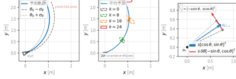
図 42: 線形 Kalman フィルタの共分散予測を差動二輪の非線形姿勢予測へ接続する幾何。左はオドメトリによる円弧状の平均姿勢予測と初期方位のずれによる終点差、中央は局所ヤコビアンで伝搬した 2\sigma 共分散楕円、右は F_k の方位列が前進距離に比例した横方向感度を表すことを示している。
