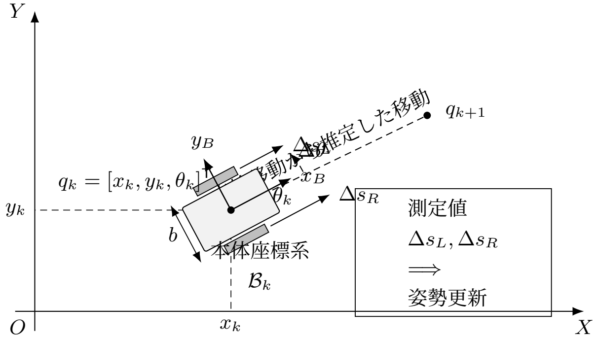
図 8: 差動二輪ロボットの上面図とオドメトリ更新。左右車輪の移動量から、世界座標系における位置 (x_k, y_k) と向き \theta_k を更新する。
