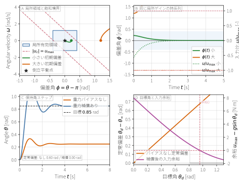
図 46: 局所線形フィードバックとモデルを使う補償の視覚的検証。上段は、同じ倒立振子の局所ゲインでも、小さい初期偏差は局所有効領域内で収束し、大きい初期偏差は入力飽和境界に張り付いて接線モデルの予測から外れることを示す。下段は、保持角を変えたとき、重力バイアスを入れない PD 制御には定常偏差が残る、重力補償を入れると目標角が平衡条件に入る一方で、必要トルクが入力上限に近づくほど余裕が消えることを示す。ただし、この図は表示したモデル、ゲイン、飽和上限の数値例であり、モデル誤差、摩擦、センサ遅れ、未表示の安全制約がある場合の安定性までは保証しない。
