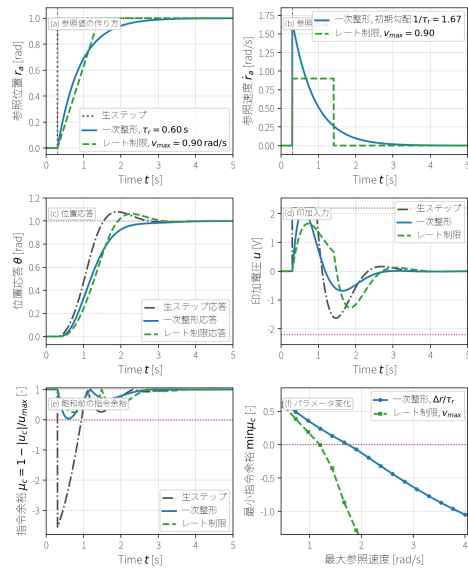
図 17: DC モータ位置サーボに対する参照値整形とレート制限の比較。生ステップは位置目標を瞬時に変えるため、飽和前の電圧指令が上限を大きく越える。一次整形は時定数 \tau_r で参照速度を有限にし、レート制限は v_{max} で参照速度そのものを制限する。下段右は最大参照速度を変えたときの最小指令余裕であり、速い参照ほど余裕が減ることを表している。
