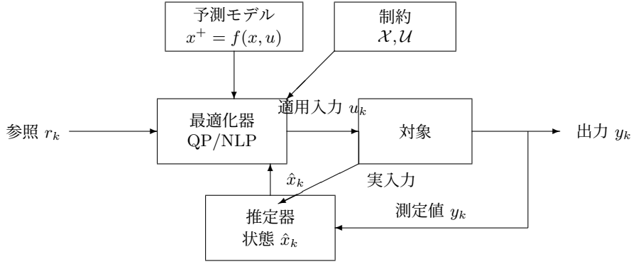
図 51: MPC の閉ループ構造。参照、推定状態、予測モデル、制約集合から最適化問題を作り、解かれた入力列の先頭だけを対象へ適用し、測定出力で次の時刻に解き直す。
