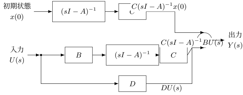
図 7: 状態空間モデルから出力 Y(s) へ至る三つの信号経路。初期状態は自然応答を作り、入力 U(s) は B と (sI - A)^{-1} と C を通る経路、および直達行列 D の経路を通して出力で加算される。
