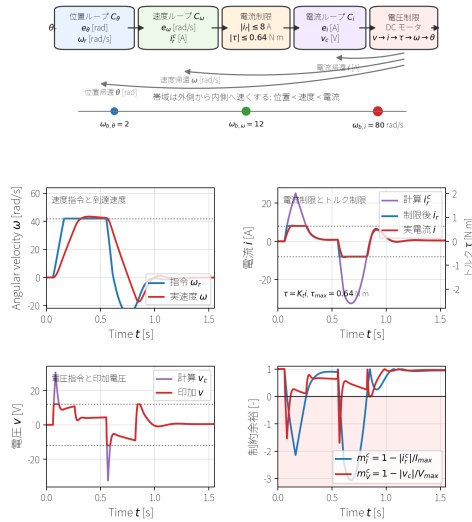
図 18: DC モータ位置サーボのカスケード構成と電流・電圧限界。上段は位置、速度、電流の三つのループを外側から内側へ配置し、帯域幅を \omega_{b,\theta} = 2 \text{ rad/s} 、 \omega_{b,\omega} = 12 \text{ rad/s} 、 \omega_{b,i} = 80 \text{ rad/s} の順に速くした例である。下段は R = 1.0 \Omega 、 L = 0.050 \text{ H} 、 K_t = K_e = 0.08 、 J = 0.003 \text{ kg m}^2 、 b = 0.002 \text{ N m s/rad} 、 I_{\max} = 8 \text{ A} 、 V_{\max} = 12 \text{ V} としたシミュレーションで、速度指令、電流指令、印加電圧、制約余裕を同じ時間軸で示す。電流指令 i_r^c と電圧指令 v_c の余裕が 0 を下回る時間帯では、外側ループが要求したトルク変化を内側ループが実現できない。
