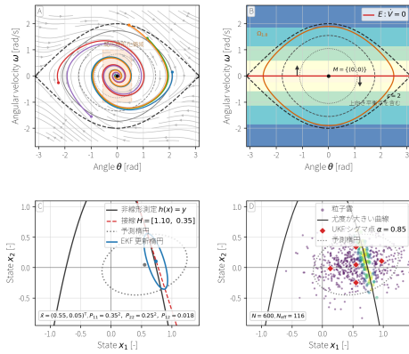
図 45: 非線形位相図、Lyapunov 準位集合、局所線形化領域、EKF の線形化楕円、UKF シグマ点、粒子雲の対応。上段は減衰係数 0.35 の正規化振子で、 V = 2 が上向き平衡点を通る境界になる。下段は h(x) = x_1^2 + 0.35x_2 、 y = 0.55 、 R = 0.08^2 の測定更新で、接線近似とサンプル表現の違いを示している。
