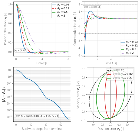
図 34: 二重積分器に対する LQR と Kalman フィルタの調整例。上段は入力重み R_u による状態応答と入力指令の変化であり、入力限界を点線で示している。左下は有限ホライズンの後退リカッチ再帰が定常解へ近づく様子である。右下は予測後の誤差共分散楕円が位置測定によって更新される様子であり、測定ノイズ分散 R_v が小さいほど測定方向の不確かさが強く縮む。
