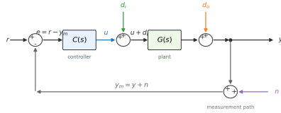
図 13: 目標値 r 、制御器 C 、制御対象 G 、入力外乱 d_i 、出力外乱 d_o 、測定ノイズ n 、制御器出力 u 、出力 y を含む閉ループの信号経路。入力外乱 d_i は対象入力側に加わるため GS の経路で y を動かし、制御器出力 u にも反作用を生む。出力外乱 d_o は対象後段で y に直接加わり、感度 S で抑えられる。測定ノイズ n は実出力を直接変えず、測定値 y_m = y + n を通じて -T と -CS の経路に入る。 u を同時に確認しないと、出力偏差が小さい条件でもアクチュエータ飽和やノイズ増幅を検出できない。
