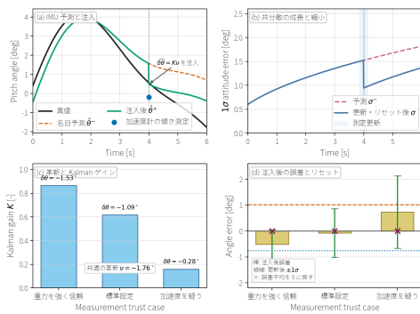
図 44: ESKF の 1 次元姿勢更新トレース。ジャイロ積分で名目姿勢がドリフトし、同時に姿勢共分散が増える。加速度計から得た傾き測定の革新で小角度誤差 \delta\theta を推定し、名目姿勢へ注入してから誤差平均を 0 へリセットする。測定を強く信頼すると加速度外乱にも寄りやすく、測定を疑うとジャイロドリフトが残りやすい。
