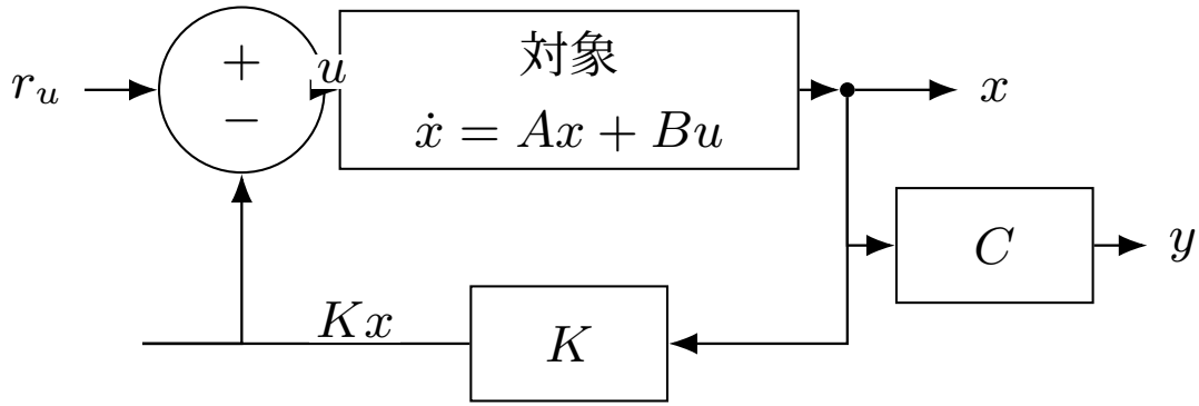
図 30: 状態フィードバック u = -Kx + r_u の信号経路。参照入力 r_u 、制御入力 u 、状態 x 、出力 y 、および Kx の負帰還経路を分けて示している。
