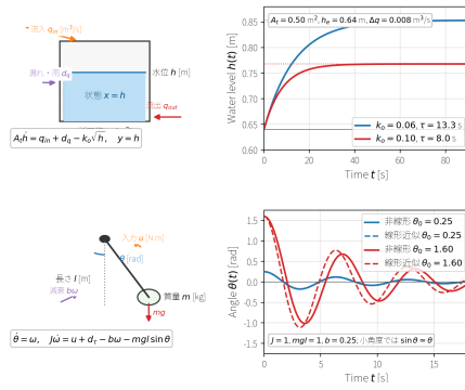
図 6: タンク水位モデルと単振りモデルの構造。タンクでは体積保存則と流出構成則から水位の状態方程式が得られ、流出係数 k_o を変えると線形化後の時定数と定常水位変化が同時に変わる。単振りではトルク、重力、粘性減衰から角度と角速度の状態方程式が得られ、小角度では線形近似と非線形応答が一致しやすいが、大振幅では周期と振幅がずれる。
