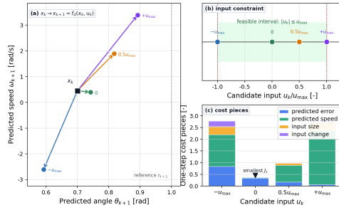
図 23: 性能指標と Pareto 図から作ったスカラー評価を、一段先の入力選択として読むための橋渡し図。現在状態 x_k 、候補入力 u_k 、予測された次状態 x_{k+1} 、入力制約 |u_k| \leq u_{\max} 、および偏差・速度・入力・入力変化の評価成分を同時に示している。この図は性能指標と Pareto 採点から有限ホライズンの見方へ移る一段の可視化であり、LQR や MPC の導出ではない。
