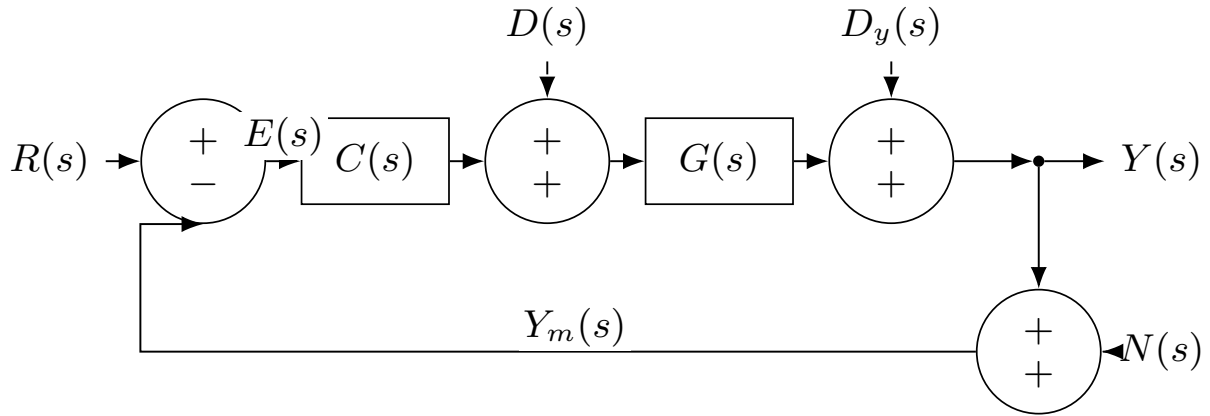
図 11: 目標値、制御器、対象、外乱、測定ノイズを含む負帰還ブロック線図
