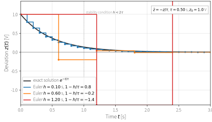
図 4: \dot{z} = -z/\tau , \tau = 0.50 s に陽的 Euler 法を適用した応答。刻み幅 h によって連続時間の減衰をどの程度再現できるかと、数値更新の安定性が変わる。
