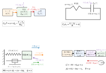
図 5: 物理法則から状態方程式へ進む標準例。熱収支では内部エネルギーの蓄積、RC 回路では電荷の蓄積、質量ばねダンパ系では位置と速度、DC モータでは電流、角速度、角度を状態として残す。各パネルは入力、外乱、代表パラメータ、状態の単位を対応させ、保存則または運動方程式から \dot{x} = f(x, u, d, p) へ整理する起点を示している。
