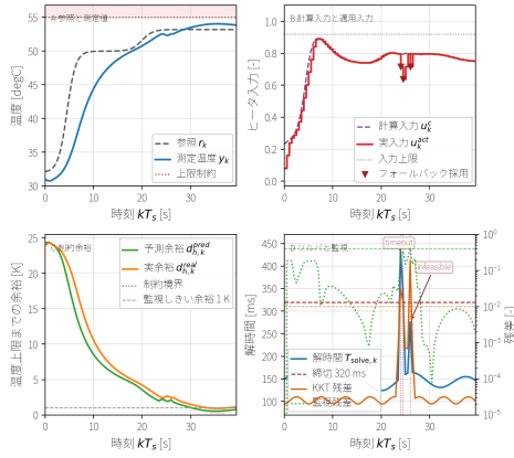
図 56: 制約付き温度制御を用いた閉ループ実装検証ログの例。参照と測定温度、計算入力と実入力、予測余裕と実余裕、解時間、KKT 残差、監視残差を同じ時刻列で比較している。
