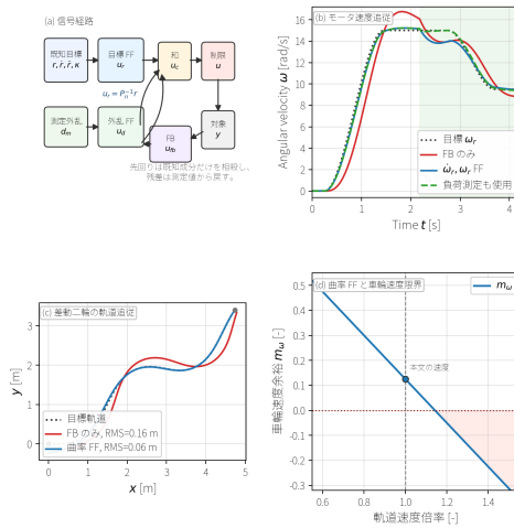
図 20: 速度・加速度フィードフォワード、曲率フィードフォワード、測定外乱補償の役割。上段左は、既知目標と測定外乱から先回り入力を作り、残差をフィードバックで戻す信号経路である。上段右は DC モータ速度追従で、 \dot{\omega}_r と \omega_r から作る電流を加えると立上り遅れが減り、負荷トルク測定 \tau_{L,m} も使うと負荷投入後の速度低下がさらに小さくなる。下段左は差動二輪ロボットの軌道追従で、曲率フィードフォワードを入れると曲がり始めの横偏差が減る。下段右は軌道速度倍率を上げたときの車輪速度余裕 m_{\omega} で、曲率が高い軌道ほど外側車輪の上限が追従可能性を決める。
