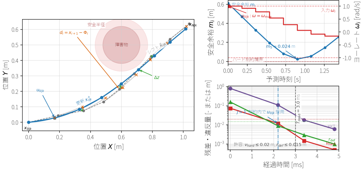
図 54: 直接多重射撃法で見た NMPC のメッシュ、後退ホライズン、ソルバ監視量。左はシフト後の節点 \bar{x}_{i|k} 、区間積分 \Phi_i(\bar{x}_{i|k}, \bar{u}_{i|k}) 、欠陥 d_i 、RTI ステップ \Delta z 、更新後の予測節点 x_{i|k}^+ を同じ平面上に重ねる。右上は障害物安全半径に対する状態余裕 m_i とヨーレート入力 \omega_i を示し、先頭入力 u_{0|k} が入力上限で能動になっていることを示す。右下は KKT 停留残差、ハード制約違反 v_{hard} 、欠陥残差 r_{def} 、締切 T_{dead} を同じサンプルの採用判定として並べる。
