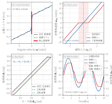
図 19: 摩擦・不感帯・バックラッシの低速測定曲線と補償例。左上は静止摩擦帯と Coulomb 摩擦を含む必要トルク、右上は不感帯を持つ電圧-角速度特性と逆向きの電圧補償、左下は往復掃引で得られるバックラッシ曲線と接触側を選ぶ角度補償、右下は反転を含む負荷角追従の補償前後である。補償後も反転直後の残差は残り、これはすきまを詰める時間と摩擦変動が残るためである。
