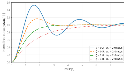
図 10: \omega_n = 2 \text{ rad/s} を固定し、減衰比 \zeta を変えた標準二次系の単位ステップ応答。減衰比により振動、オーバーシュート、整定の速さが変わる。
