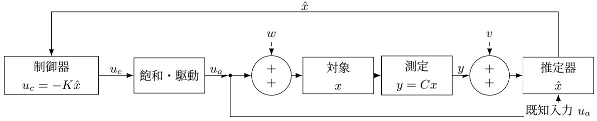
図 35: LQG 制御の信号経路。測定 y から推定器が \hat{x} を作り、制御器が入力指令 u_c を計算し、飽和や駆動系を通った実入力 u_a が対象へ入る。線形導出では u_a = u_c とみなすが、飽和がある場合は実入力を推定器の既知入力として扱う。
