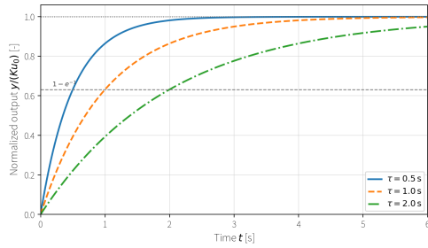
図 9: 正規化した一次遅れ応答。 y/(Ku_0) = 1 - e^{-t/\tau} において時定数 \tau だけを変えており、各曲線は t = \tau で 1 - e^{-1} に達する。
