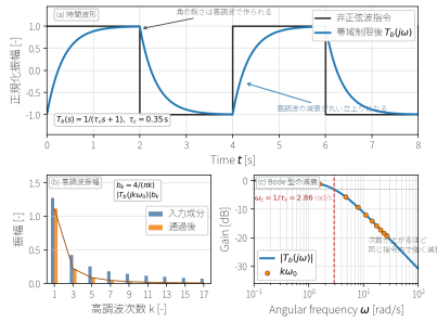
図 25: 非正弦波指令を高調波成分へ分け、一次的な閉ループ帯域 T_b(s) = 1/(\tau_c s + 1) に通したときの対応。上段は時間波形であり、方形波指令の角が帯域制限後に丸められる。左下は各奇数次高調波の入力振幅 b_k = 4/(\pi k) と通過後の振幅 |T_b(jk\omega_0)|b_k を比べる。右下は同じ T_b(j\omega) のゲインを Bode 型の減衰曲線として示し、高い次数の成分ほど折点周波数より上で強く減衰することを確認する。
