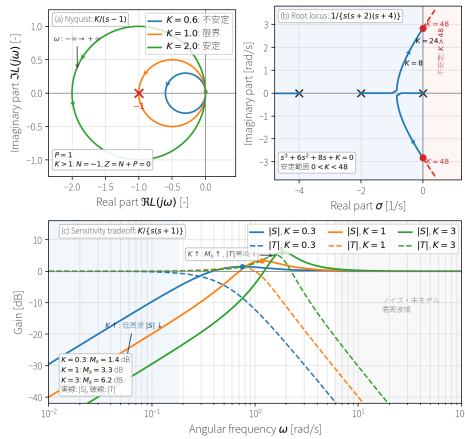
図 27: ナイキスト線図、根軌跡、感度関数を同じ周波数設計の確認図として並べた例。上左は不安定開ループ極 P = 1 を持つ L_K(s) = K/(s-1) のゲイン変化で、 K > 1 だけが点 -1 を反時計回りに 1 回囲み閉ループが安定になる。上右は三次開ループ G(s) = 1/\{s(s+2)(s+4)\} の根軌跡で、 0 < K < 48 が安定範囲、 K = 48 で虚軸を横切る。下は L_K(s) = K/\{s(s+1)\} の S と T で、ゲインを上げるほど低周波の外乱抑制は強くなるが、感度ピークと相補感度の通過帯域が増える。
