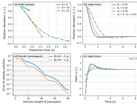
図 33: 有限ホライズン LQR における予測、重み掃引、後退リカッチ収束の例。二重積分器で予測ホライズン N を変えると、予測区間に含まれる将来偏差が変わる。入力重み R_u や位置重み q_1 を変えると、位置偏差の整定、入力努力、入力限界 \pm 2 に対する制約余裕が同時に変わる。左下は S_N = 0 から後退リカッチ再帰を始めても、ホライズンを長くすると現在時刻の P_0(N) と K_0(N) が定常解 P_\infty, K_\infty へ近づくことを示す。
