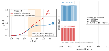
図 37: 差動駆動ロボットの真の軌跡とエンコーダオドメトリのずれ、および 1 サンプル内の左右エンコーダパルスの例。右車輪が床に対して滑ると、エンコーダは車輪の回転を数え続けるため、オドメトリは実際の床上移動より大きい右車輪距離を積分する。
