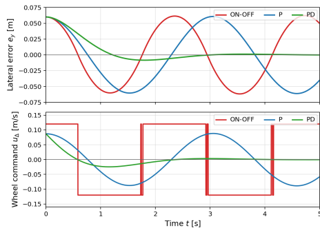
図 12: ライントレースロボットの横偏差に対する ON-OFF、P、PD 制御の比較。上段は横偏差 e_y 、下段は左右車輪速度差指令 u_\Delta = v_L - v_R を示す。ON-OFF 制御は符号切替により中心付近で指令が反転し、P 制御は連続指令に変わるが減衰を持たず、PD 制御は横偏差の変化率を使って振動を減らす。
