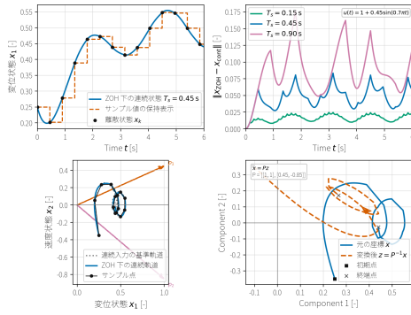
図 28: 二状態モデルにおける状態遷移、ZOH 離散化、サンプリング周期、座標変換の関係。左上は ZOH 入力のもとで連続状態が曲線として動き、離散モデルはサンプル時刻の点列を与えることを示す。右上は滑らかな入力を ZOH 入力で近似したときの状態誤差であり、 T_s が大きいほど保持入力の粗さが状態へ残る。左下は同じ現象を状態平面上の軌道として表し、右下は P = \begin{bmatrix} 1 & 1 \\ 0.45 & -0.85 \end{bmatrix} とした x = Pz による別の基底で同じ軌道を表示している。
