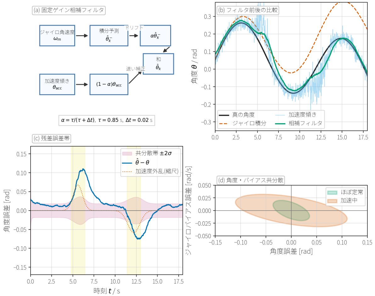
図 41: ジャイロ積分、加速度計傾き、相補フィルタ、残差不確かさの関係。左上は固定係数の信号経路、右上はドリフトと加速度外乱を含む測定の前後比較、左下はフィルタ後の残差と共分散帯、右下は角度誤差とジャイロバイアス誤差の楕円表示である。加速区間では加速度計の見かけの傾きが悪化し、固定係数のままでは信頼度の変化を推定器の内部状態として保持できない。
