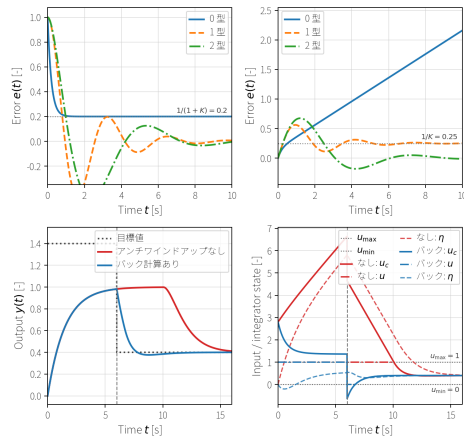
図 15: 系の型による定常偏差と、飽和時の PI 制御におけるアンチwindアップ効果。上段は L_0(s) = 4/(s+1) 、 L_1(s) = 4/\{s(s+1)\} 、 L_2(s) = 4(s+1)/\{s^2(s+4)\} の単位負帰還を同じ入力と比較し、型が上がると追従できる基準入力の次数が一つずつ上がることを示す。下段は P(s) = 1/(1.5s+1) 、 K_P = 2.0 、 K_I = 1.5 、 0 \leq u \leq 1 の PI 制御で、計算入力 u_c 、適用入力 u 、飽和限界、積分状態 \eta を比較し、バック計算が飽和中の積分状態を入力制約に合わせて戻すことを示す。
