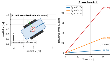
図 39: 差動二輪ロボットに固定した IMU の機体軸と、一定ジャイロバイアスによるヨー角誤差の蓄積。左図では IMU が機体系 \{B\} に固定され、 z_B 軸まわりの角速度を測る。右図では T_s = 0.01\text{ s} でジャイロを積分し、バイアスが 0.1^\circ/\text{s} 、 0.5^\circ/\text{s} 、 1.5^\circ/\text{s} のとき、誤差がそれぞれ 60 s 後に 6^\circ 、 30^\circ 、 90^\circ へ達することを示している。
