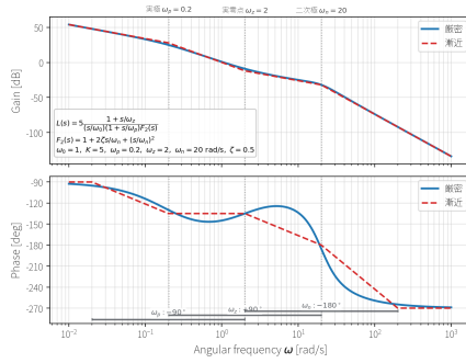
図 26: 正規化された開ループ L(s) のボード線図。0.2 rad/s の実極でゲイン傾きが下がり、2 rad/s の実零点で戻り、20 rad/s の二次極でさらに低下する。破線の漸近線と実線の厳密線図を比べると、折点近傍の誤差と位相遷移を確認できる。
