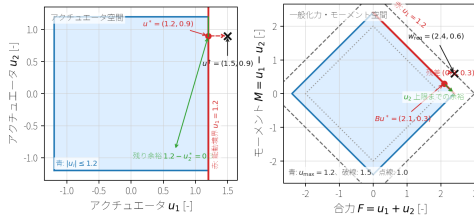
図 55: 制御配分の飽和幾何。左はアクチュエータ空間で、制約なし配分 u^\dagger = (1.5, 0.9)^\top が上限 u_1 = 1.2 の外へ出ることを示す。右は同じ上限制約を合力 F とモーメント M の空間へ写した図であり、要求 w_{\text{req}} = (2.4, 0.6)^\top は実現可能領域の外にある。飽和後の実現値は Bu^* = (2.1, 0.3)^\top で、赤い矢印が残差、緑の線分が第二入力側に残る余裕を表す。
