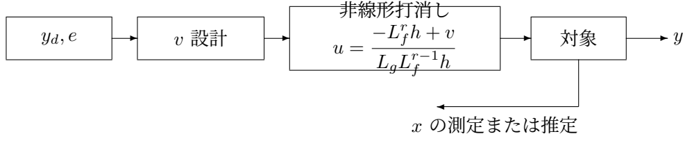
図 47: 入出力線形化の信号経路。この図は、追従誤差から仮想入力 v を作り、状態 x に依存する非線形項を入力変換で打ち消すと、出力側だけが y^{(r)} = v へ置き換わることを示す。ただし、零ダイナミクスの安定性、状態推定誤差、モデル誤差、入力飽和の可否まではこの図だけでは保証しない。
