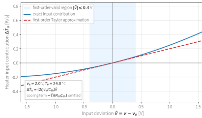
図 3: T_a = 20^\circ\text{C} 、 R_{th} = 2.0\text{ K/W} 、 C_{th} = 10\text{ J/K} 、 \eta = 0.5\text{ W/V}^2 、 v_e = 2.0\text{ V} の動作点におけるヒータ入力寄与と一次 Taylor 近似。偏差が小さい範囲では一次近似を使いやすい。
