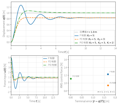
図 16: 質量ばねダンパ系に対する P、PD、PID 候補設計の比較。対象は m = 1 \text{ kg} 、 c = 1 \text{ Ns/m} 、 k = 1 \text{ N/m} 、目標値は r = 1 \text{ m} である。PD 制御は速度フィードバックで振動を抑え、PID 制御は積分状態で定常偏差を減らす、操作力の使い方も変わる。
