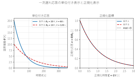
図 1: ケース A ( \theta_0 = 20 \text{ K} , \tau = 60 \text{ s} ) とケース B ( \theta_0 = 10 \text{ K} , \tau = 120 \text{ s} ) の一次遅れ応答。左は次元つきの時間 t と温度偏差 \theta で描いた図であり、初期偏差と時定数が異なるため曲線の高さと減衰速度が異なる。右は \xi = t/\tau と x = \theta/\theta_0 で正規化した図であり、両者が x = e^{-\xi} に重なるため、単位や実験スケールを越えて同じ減衰過程として比較できる。
