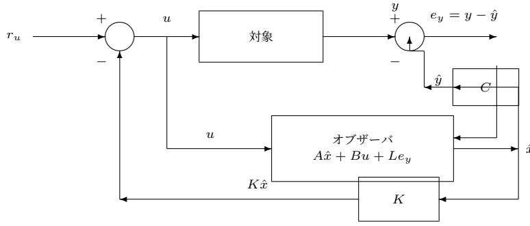
図 16: 推定状態を用いる状態フィードバックと Luenberger オブザーバの信号経路。対象とオブザーバには同じ制御入力 u が入り、測定値 y と推定出力 \hat{y} = C\hat{x} の差 e_y が推定誤差を修正する。
