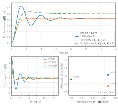
図 13: 質量ばねダンパ系に対する P、PD、PID 候補設計の比較。対象は m = 1 \text{ kg} 、 c = 1 \text{ N s/m} 、 k = 1 \text{ N/m} 、目標値は r = 1 \text{ m} である。PD 制御は速度フィードバックで振動を抑え、PID 制御は積分状態で定常偏差を減らす、操作力の使い方も変わる。
