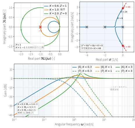
図 11: ナイキスト線図、根軌跡、感度関数を同じ周波数設計の確認図として並べた例。上左は不安定開ループ極 P = 1 を持つ L_K(s) = K/(s-1) のゲイン変化で、 K > 1 だけが点 -1 を反時計回りに 1 回囲み閉ループが安定になる。上右は三次開ループ G(s) = 1/\{s(s+2)(s+4)\} の根軌跡で、 0 < K < 48 が安定範囲、 K = 48 で虚軸を横切る。下は L_K(s) = K/\{s(s+1)\} の S と T で、ゲインを上げるほど低周波の外乱抑制は強くなるが、感度ピークと相補感度の通過帯域が増える。
