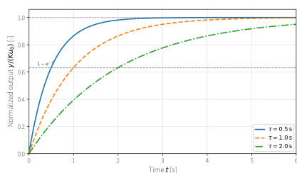
図 6: 正規化した一次遅れ応答。 y/(Ku_0) = 1 - e^{-t/\tau} において時定数 \tau だけを変えており、各曲線は t = \tau で 1 - e^{-1} に達する。
