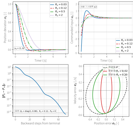
図 18: 二重積分器に対する LQR と Kalman フィルタの調整例。上段は入力重み R_u による状態応答と入力指令の変化であり、入力限界を点線で示している。左下は有限ホライズンの後退りカッチ再帰が定常解へ近づく様子である。右下は予測後の誤差共分散楕円が位置測定によって更新される様子であり、測定ノイズ分散 R_v が小さいほど測定方向の不確かさが強く縮む。
