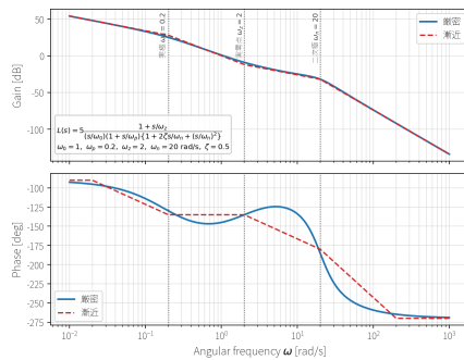
図 10: 正規化された開ループ L(s) のボード線図。0.2 rad/s の実極でゲイン傾きが下がり、2 rad/s の実零点で戻り、20 rad/s の二次極でさらに低下する。破線の漸近線と実線の厳密線図を比べると、折点近傍の誤差と位相遷移を確認できる。
