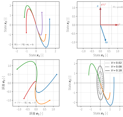
図 17: 二状態モデル A = \begin{bmatrix} 0 & 1 \\ -2 & -3 \end{bmatrix} 、 b = \begin{bmatrix} 0 & 1 \end{bmatrix}^T 、 C = \begin{bmatrix} 1 & 0 \end{bmatrix} に対する状態空間の幾何。左上は K = \begin{bmatrix} 18 & 6 \end{bmatrix} による閉ループ軌道、右上は可制御方向 B , AB と可観測方向 C^T , A^T C^T 、左下は L = \begin{bmatrix} 10 & 10 \end{bmatrix}^T による推定誤差軌道、右下は A - bK に対する V = x^T P x のレベル集合を示す。
