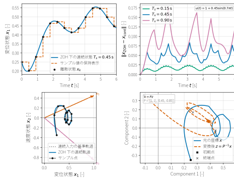
図 14: 二状態モデルにおける状態遷移、ZOH 離散化、サンプリング周期、座標変換の関係。左上は ZOH 入力のもとで連続状態が曲線として動き、離散モデルはサンプル時刻の点列を与えることを示す。右上は滑らかな入力を ZOH 入力で近似したときの状態誤差であり、 T_s が大きいほど保持入力の粗さが状態へ残る。左下は同じ現象を状態平面上の軌道として表し、右下は P = \begin{bmatrix} 1 & 1 \\ 0.45 & -0.85 \end{bmatrix} とした x = Pz による別の基底で同じ軌道を表示している。
