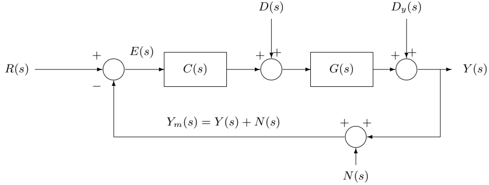
図 8: 目標値、制御器、対象、外乱、測定ノイズを含む負帰還ブロック線図
