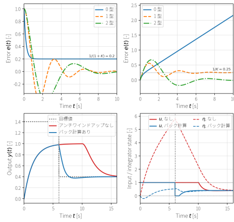
図 12: 系の型による定常偏差と、飽和時の PI 制御におけるアンチwindアップ効果。上段は L_0(s) = 4/(s+1) 、 L_1(s) = 4/\{s(s+1)\} 、 L_2(s) = 4(s+1)/\{s^2(s+4)\} の単位負帰還を同じ入力と比較し、型が上がると追従できる基準入力の次数が一つずつ上がることを示す。下段は P(s) = 1/(1.5s+1) 、 K_P = 2.0 、 K_I = 1.5 、 0 \leq u \leq 1 の PI 制御で、バック計算が飽和中の積分状態を入力制約に合わせて戻すことを示す。
