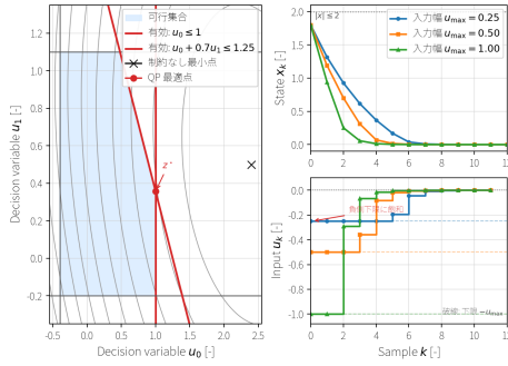
図 23: MPC と QP の制約を視覚化した例。左は決定変数 z = (u_0, u_1) の可行集合、二次目的関数の等高線、制約なし最小点、制約付き最適点を示し、赤い境界が能動制約である。右は x_{k+1} = 0.8x_k + 0.5u_k 、 N = 8 、初期値 x_0 = 1.8 の閉ループで、入力上下限 [-u_{\max}, u_{\max}] を変えたときの状態と適用入力を比較している。入力幅が狭いほど負方向の下限 -u_{\max} に張り付き、状態の減衰が遅くなる。
