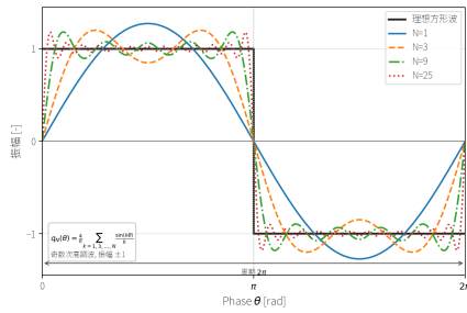
図 9: 周期 2\pi 、振幅 \pm 1 に正規化した方形波と、奇数次高調波 k = 1, 3, \dots, N だけを N = 1, 3, 9, 25 で打ち切ったフーリエ部分和。高い奇数次高調波ほど不連続点近傍の鋭い立上りを作るため、帯域制限をもつ制御対象や閉ループでは方形波指令や急な外乱が丸められ、帯域付近の位相遅れや共振が過渡応答として現れやすい。
