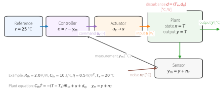
図 1: 熱系における参照信号、制御器、アクチュエータ、対象、センサ、外乱、ノイズの入る位置。外乱は対象の状態を変え、ノイズはセンサ測定値に加わる。
