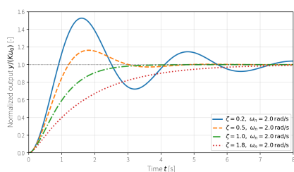
図 7: \omega_n = 2 \text{ rad/s} を固定し、減衰比 \zeta を変えた標準二次系の単位ステップ応答。減衰比により振動、オーバーシュート、整定の速さが変わる。
