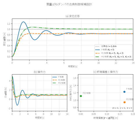
図 14: 質量ばねダンパ系に対する P、PD、PID 候補設計の比較。対象は m = 1 \text{ kg} 、 c = 1 \text{ Ns/m} 、 k = 1 \text{ N/m} 、目標値は r = 1 \text{ m} である。PD 制御は速度フィードバックで振動を抑え、PID 制御は積分状態で定常偏差を減らす、操作力の使い方も変わる。
