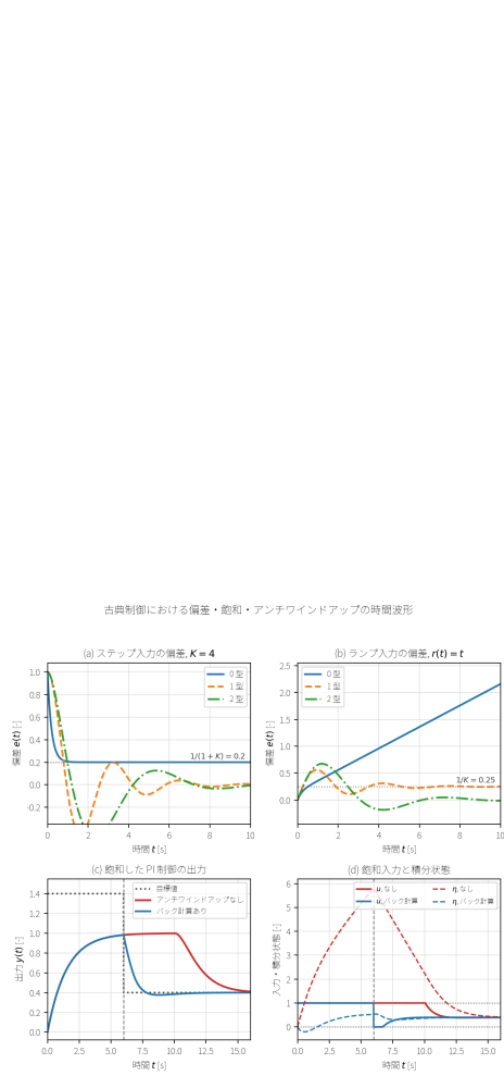
図 13: 系の型による定常偏差と、飽和時の PI 制御におけるアンチwindアップ効果。上段は L_0(s) = 4/(s+1) 、 L_1(s) = 4/\{s(s+1)\} 、 L_2(s) = 4(s+1)/\{s^2(s+4)\} の単位負帰還を同じ入力で比較し、型が上がると追従できる基準入力の次数が一つずつ上がることを示す。下段は P(s) = 1/(1.5s+1) 、 K_P = 2.0 、 K_I = 1.5 、 0 \leq u \leq 1 の PI 制御で、バック計算が飽和中の積分状態を入力制約に合わせて戻すことを示す。
