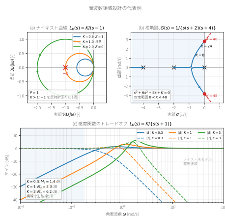
図 12: ナイキスト線図、根軌跡、感度関数を同じ周波数設計の確認図として並べた例。上左は不安定開ループ極 P=1 を持つ L_K(s) = K/(s-1) のゲイン変化で、 K > 1 だけが点 -1 を反時計回りに 1 回囲み閉ループが安定になる。上右は三次開ループ G(s) = 1/\{s(s+2)(s+4)\} の根軌跡で、 0 < K < 48 が安定範囲、 K=48 で虚軸を横切る。下は L_K(s) = K/\{s(s+1)\} の S と T で、ゲインを上げるほど低周波の外乱抑制は強くなるが、感度ピークと相補感度の通過帯域が増える。
