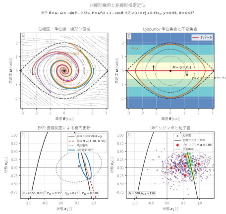
図 22: 非線形位相図、Lyapunov 準位集合、局所線形化領域、EKF の線形化楕円、UKF シグマ点、粒子雲の対応。上段は減衰係数 0.35 の正規化振子で、 V = 2 が上向き平衡点を通る境界になる。下段は h(x) = x_1^2 + 0.35x_2 、 y = 0.55 、 R = 0.08^2 の測定更新で、接線近似とサンプル表現の違いを示している。
