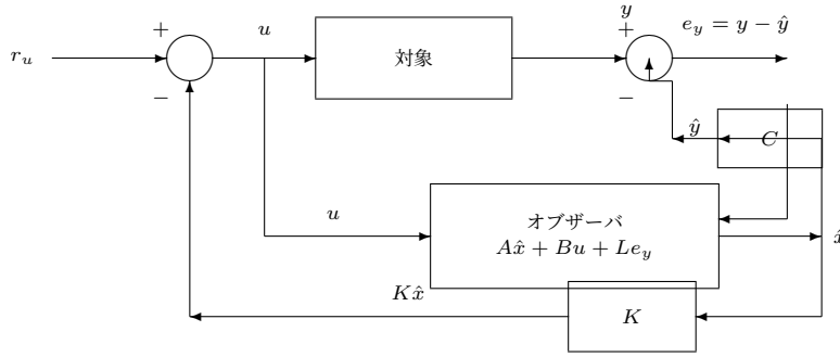
図 17: 推定状態を用いる状態フィードバックと Luenberger オブザーバの信号経路。対象とオブザーバには同じ制御入力 u が入り、測定値 y と推定出力 \hat{y} = C\hat{x} の差 e_y が推定誤差を修正する。
