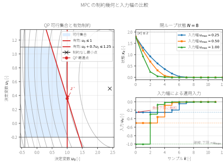
図 24: MPC と QP の制約を視覚化した例。左は決定変数 z = (u_0, u_1) の可行集合、二次目的関数の等高線、制約なし最小点、制約付き最適点を示し、赤い境界が能動制約である。右は x_{k+1} = 0.8x_k + 0.5u_k 、 N = 8 、初期値 x_0 = 1.8 の閉ループで、入力上下限 [-u_{\max}, u_{\max}] を変えたときの状態と適用入力を比較している。入力幅が狭いほど負方向の下限 -u_{\max} に張り付き、状態の減衰が遅くなる。
