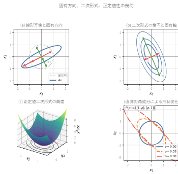
図 4: 固有方向、二次形式、正定値性の幾何的關係。左上は線形写像 A が一般の方向を曲げる一方、固有ベクトル方向では伸縮だけを与えることを示す。右上は x^T P x = \text{const.} の楕円と固有軸を対応させている。左下は正定値二次形式が原点を底とする曲面を作ることを示す。右下は非対角成分 \rho を大きくすると楕円が傾き、ある方向が強く罰せられることを示す。
