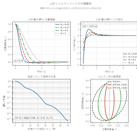
図 19: 二重積分器に対する LQR と Kalman フィルタの調整例。上段は入力重み R_u による状態応答と入力指令の変化であり、入力限界を点線で示している。左下は有限ホライズンの後退リカッチ再帰が定常解へ近づく様子である。右下は予測後の誤差共分散楕円が位置測定によって更新される様子であり、測定ノイズ分散 R_v が小さいほど測定方向の不確かさが強く縮む。
