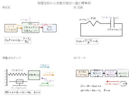
図 6: 物理法則から状態方程式へ進む標準例。熱収支では内部エネルギーの蓄積、RC 回路では電荷の蓄積、質量ばねダンパ系では位置と速度、DC モータでは電流、角速度、角度を状態として残す。各パネルは入力、外乱、代表パラメータ、状態の単位を対応させ、保存則または運動方程式から \dot{x} = f(x, u, d, p) へ整理する起点を示している。
