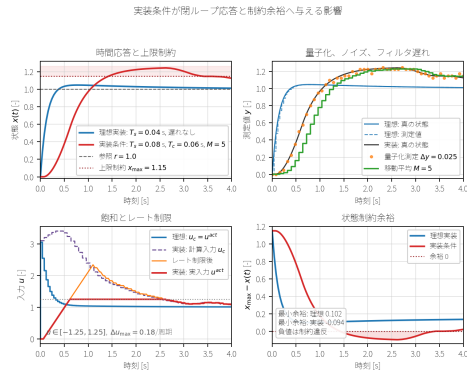
図 25: 実装条件による閉ループ応答、測定信号、実入力、状態制約余裕の変化。一次遅れ対象を同じ制御器で追従させ、理想的な離散実装と、 T_s = 0.08 [s]、計算遅れ T_c = 0.06 [s]、量子化幅 \Delta y = 0.025 、移動平均長 M = 5 、入力範囲 [-1.25, 1.25] 、レート制限 \Delta u_{\max} = 0.18/\text{周期} を含む実装を比較している。
