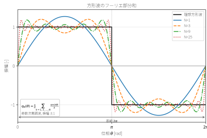
図 10: 周期 2\pi 、振幅 \pm 1 に正規化した方形波と、奇数次高調波 k = 1, 3, \dots, N だけを N = 1, 3, 9, 25 で打ち切ったフーリエ部分和。高い奇数次高調波ほど不連続点近傍の鋭い立上りを作るため、帯域制限をもつ制御対象や閉ループでは方形波指令や急な外乱が丸められ、帯域付近の位相遅れや共振が過渡応答として現れやすい。
