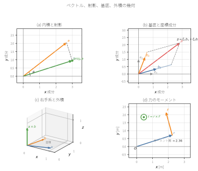
図 3: ベクトル、射影、基底、外積の幾何的關係。左上は内積が作る射影と直交成分を示す。右上は同じ点 p が標準基底と斜めの基底で異なる座標成分を持つことを示す。左下は右手系で a \times b が a と b の張る平面に垂直な向きを持つことを示す。右下は作用点ベクトル r と力 F から、回転軸まわりのモーメント \tau = r \times F が決まることを示す。
