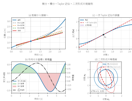
図 2: 微分、積分、Taylor 近似、二次形式を制御で使う前に確認する視覚例。左上は割線が接線へ近づく過程であり、平均変化率から微分係数へ進む極限を示す。左下は正負の変化率 r(t) を符号付き面積として足し合わせ、その累積量が時間とともに変わる様子を示す。右上は操作点 x_0 での一次 Taylor 近似と真の関数との差であり、線形化の有効範囲を示す。右下は P_1 = \begin{bmatrix} 1 & 0 \\ 0 & 1 \end{bmatrix} と P_2 = \begin{bmatrix} 3 & 1.1 \\ 1.1 & 1 \end{bmatrix} が作る x^T P x = 1, 2.25 の等高線であり、重みが多い方向ほど同じ値の楕円が狭くなる。
