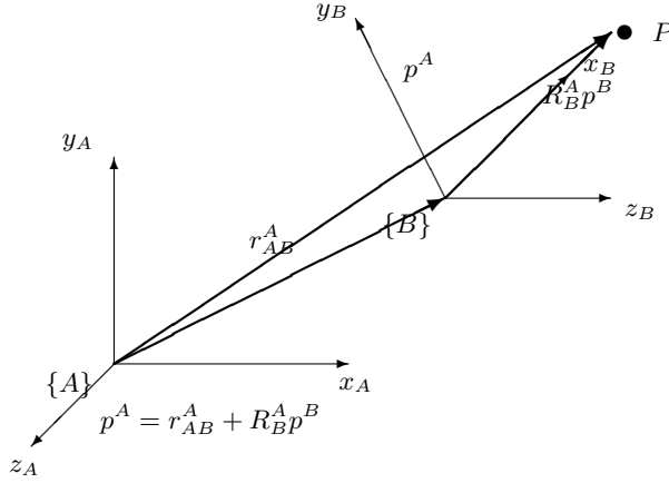
図 21: 座標系の原点移動と回転を含む点の座標変換
