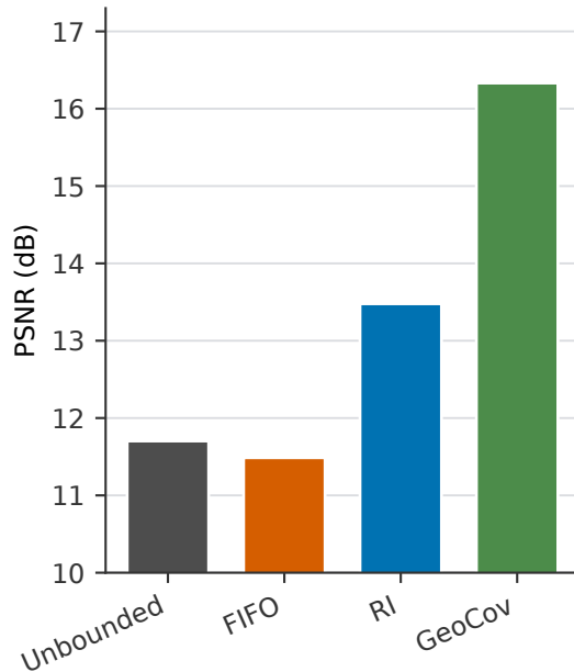
Same-video selected PSNR
