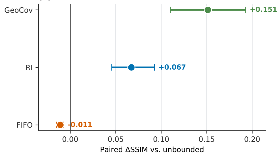
(d) The same result holds in SSIM
