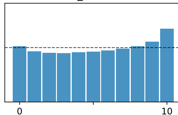
sfno_modes10
