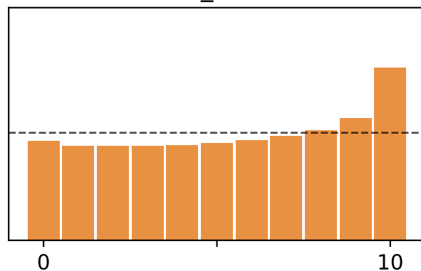
aurora_encoder
