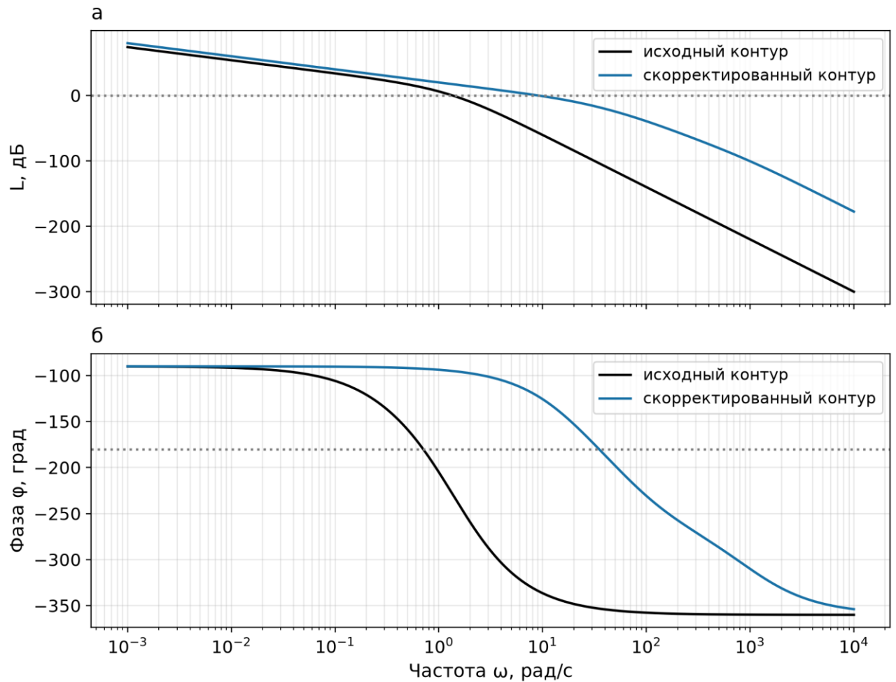
Рисунок 5 — Частотные характеристики: а – ЛАЧХ; б – фаза
