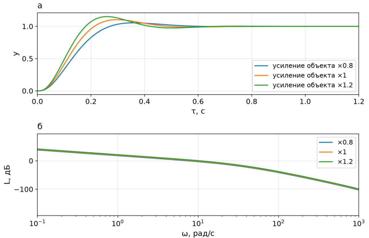
Рисунок 9 — Влияние усиления: а – переходный процесс; б – ЛАЧХ
