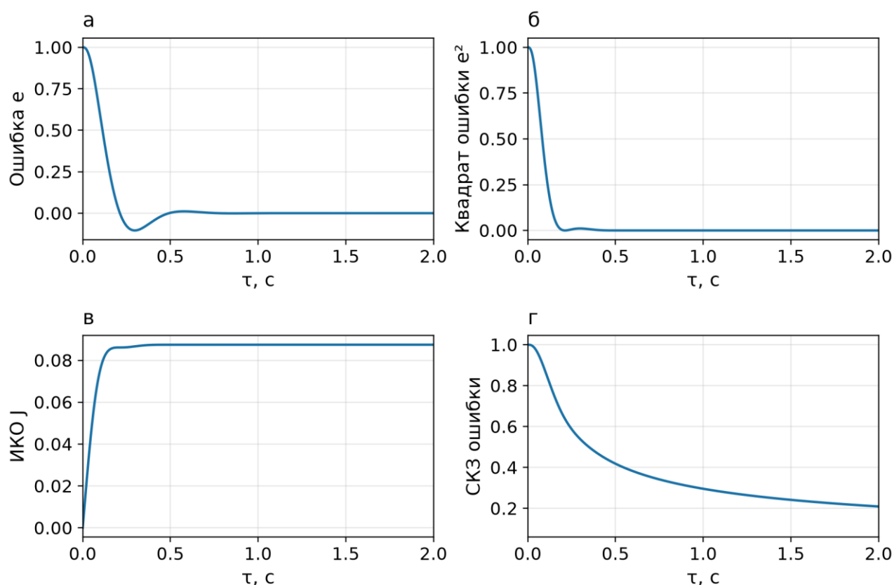
Рисунок 7 — Показатели ошибки: а – ошибка; б – её квадрат; в – ИКО; г – СКЗ
