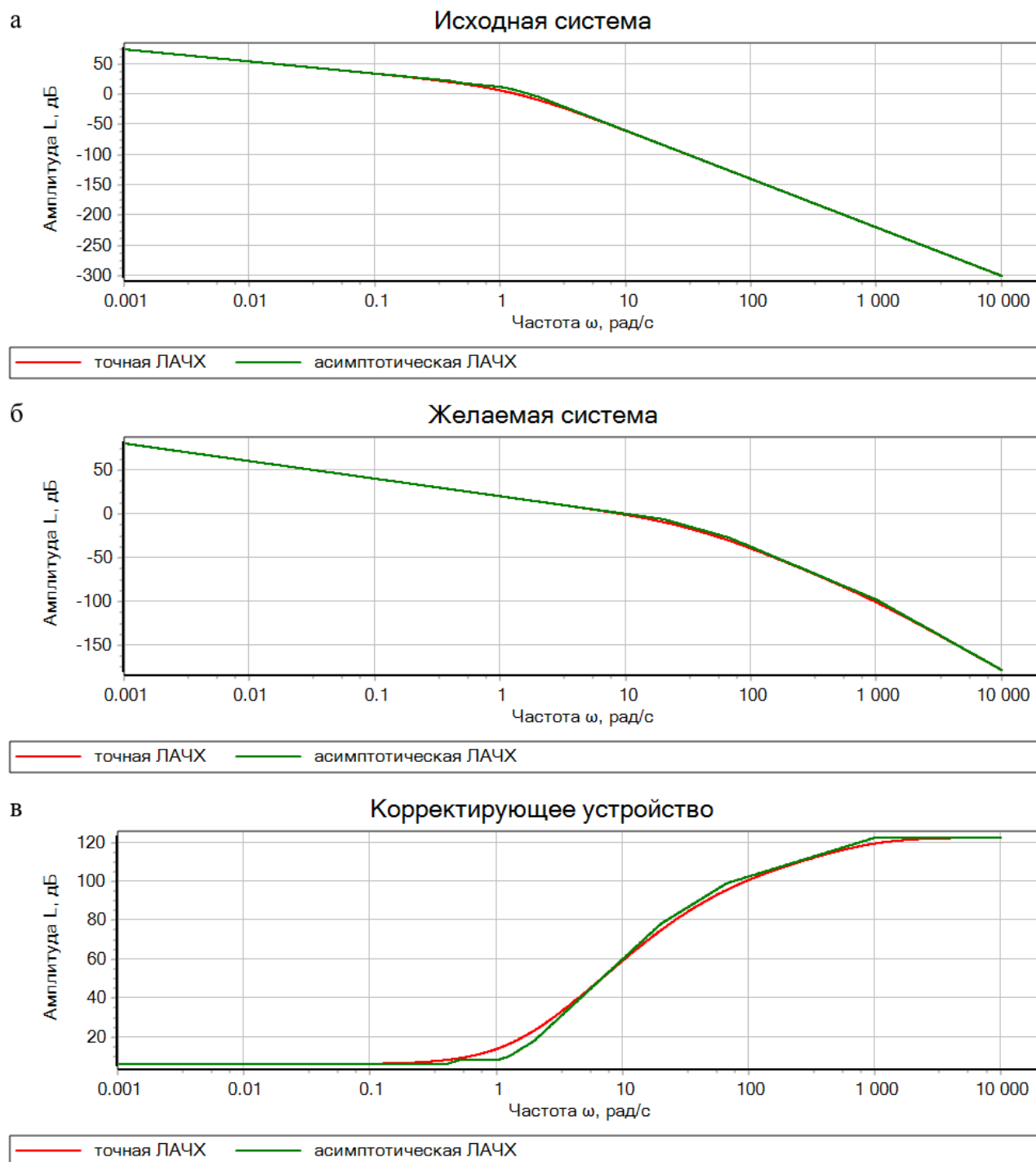
Рисунок 2 — Точные и асимптотические ЛАЧХ: а – исходная система; б – желаемая система; в – КУ
