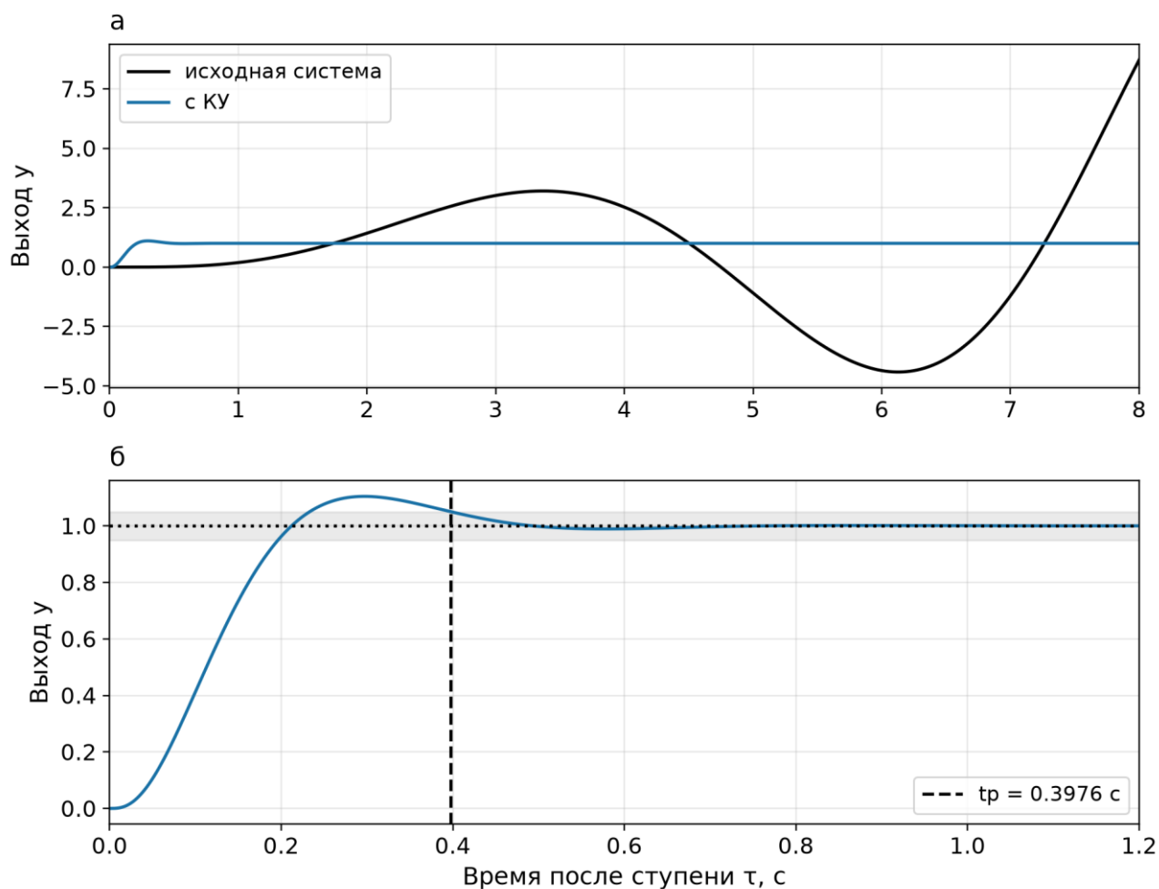
Рисунок 6 — Переходные характеристики: а – сравнение систем; б – реакция с КУ в полосе \pm 5\%
