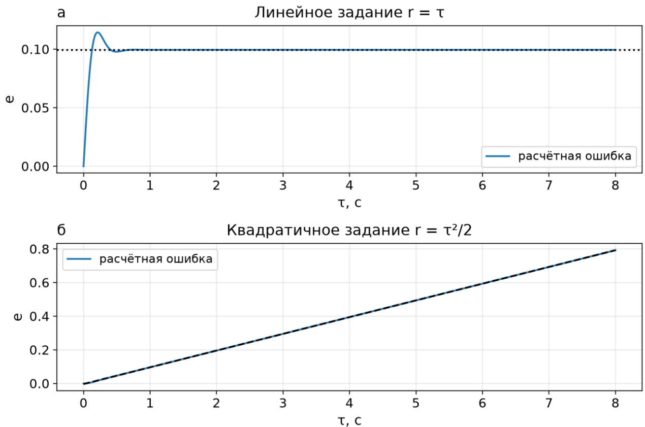
Рисунок 8 — Ошибки слежения: а – линейное задание; б – квадратичное
