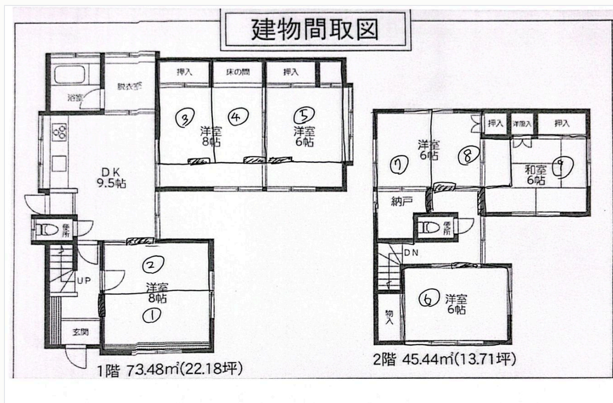
図3 9室化の割付案（①～⑨）。1階 洋8→①②、洋8+床の間→③④、洋6→⑤／2階 洋6→⑥、洋6+納戸→⑦⑧、和6→⑨
