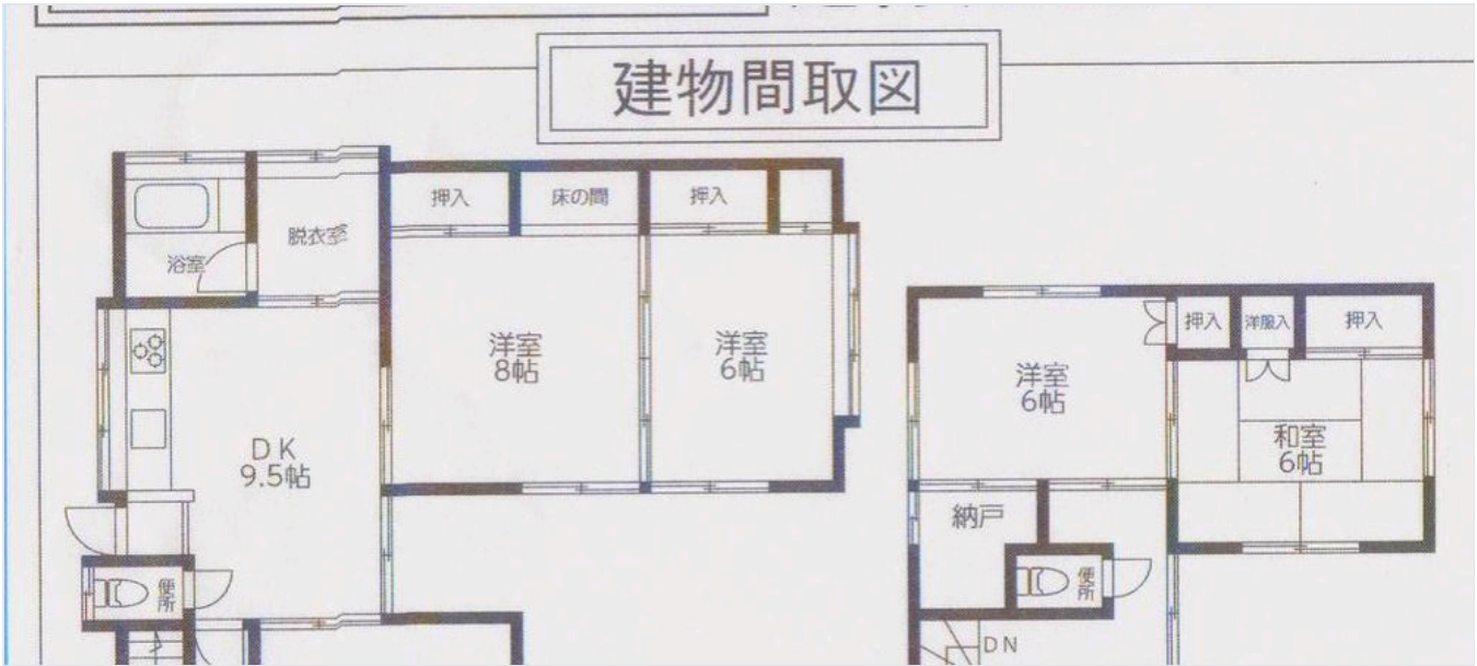
図2 現況間取図（1階73.48㎡／2階45.44㎡）と配置図（12.100×12.600、指定道路幅4.00m、間口4.20m）
