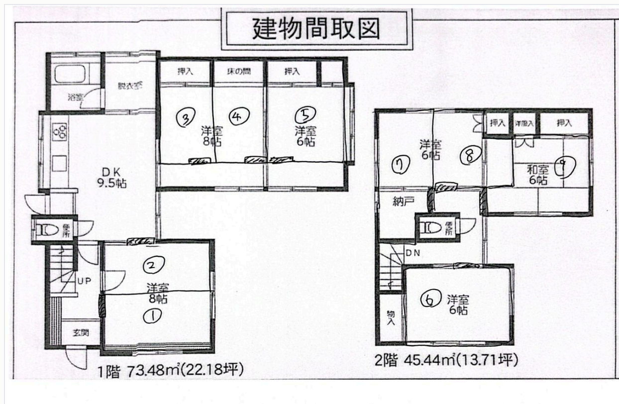
図3 9室化の割付案（①～⑨）。1階 洋8→①②、洋8+床の間→③④、洋6→⑤／2階 洋6→⑥、洋6+納戸→⑦⑧、和6→⑨
