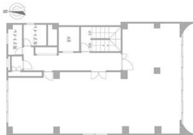
2階平面図
