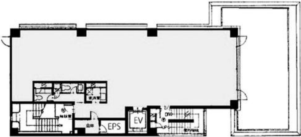
5階平面図
