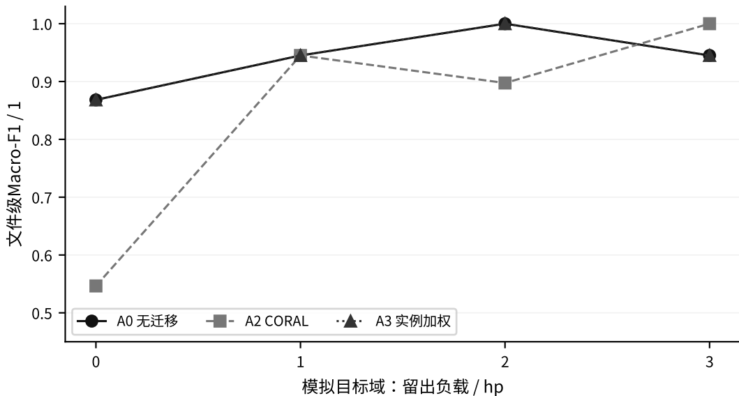
F07 无监督迁移候选在可评价模拟目标域上的表现（参数由模拟协议冻结）
