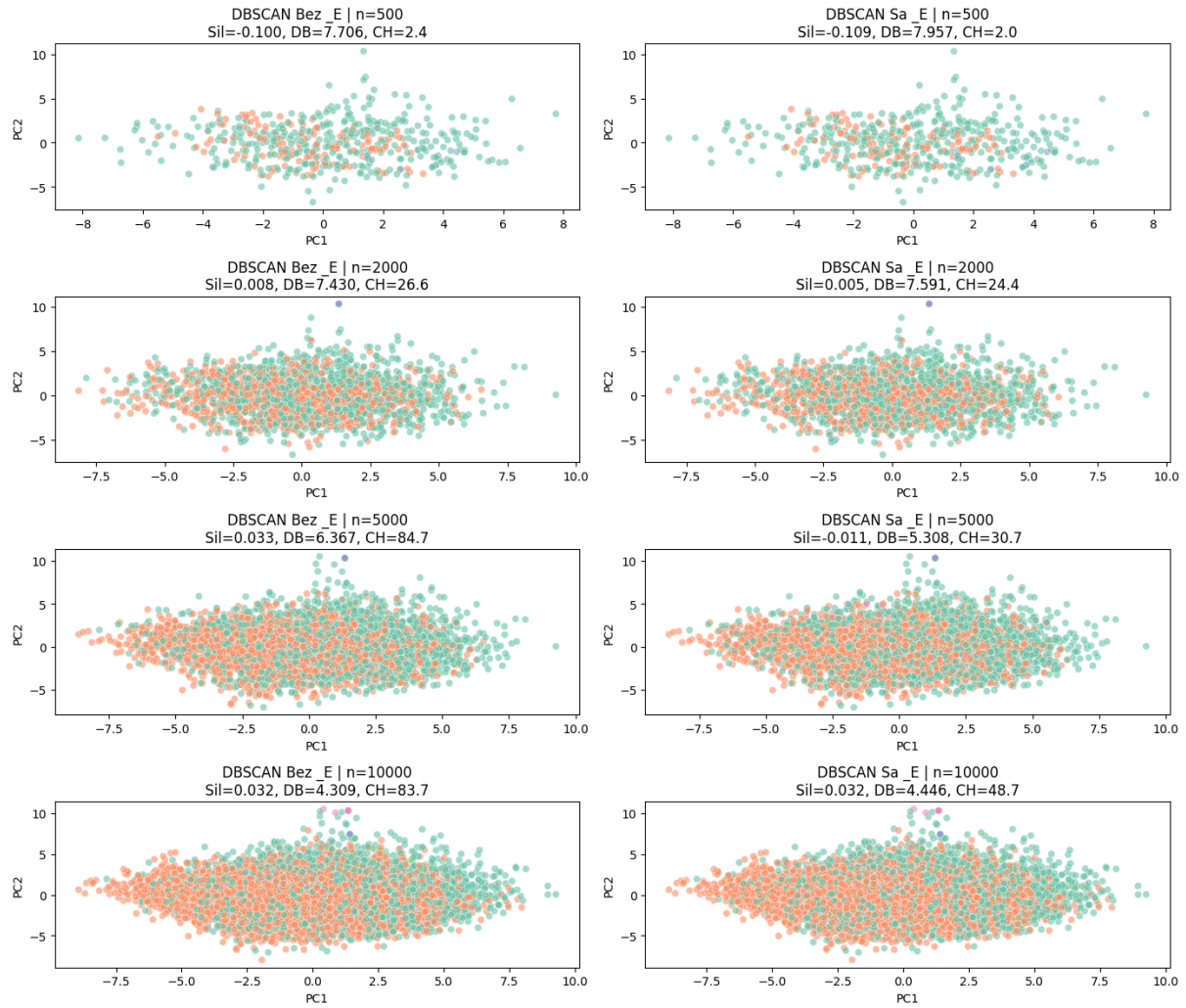
Slika 7: DBSCAN ( \epsilon = 5.5 ) za različite veličine uzorka – poređenje bez i sa vremenskim promenljivama
