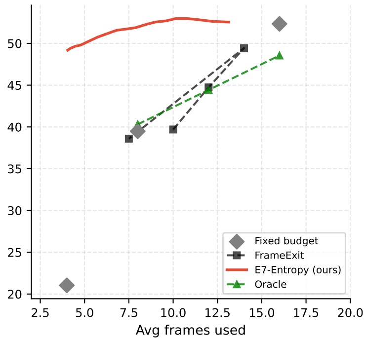
VideoMAE / SSv2
