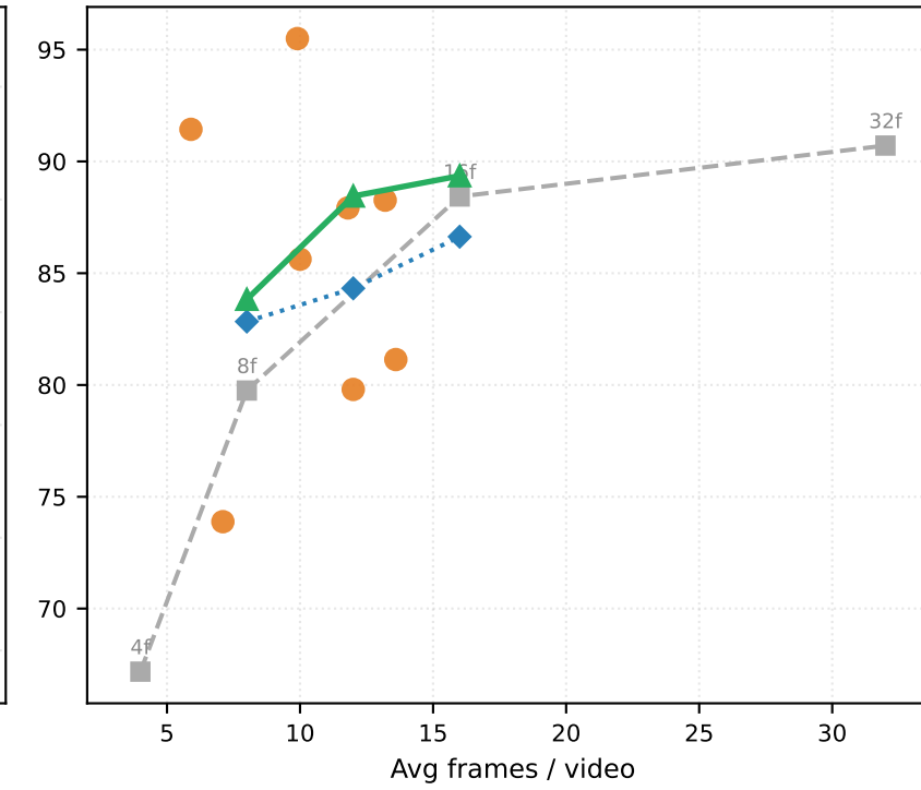
UCF101
