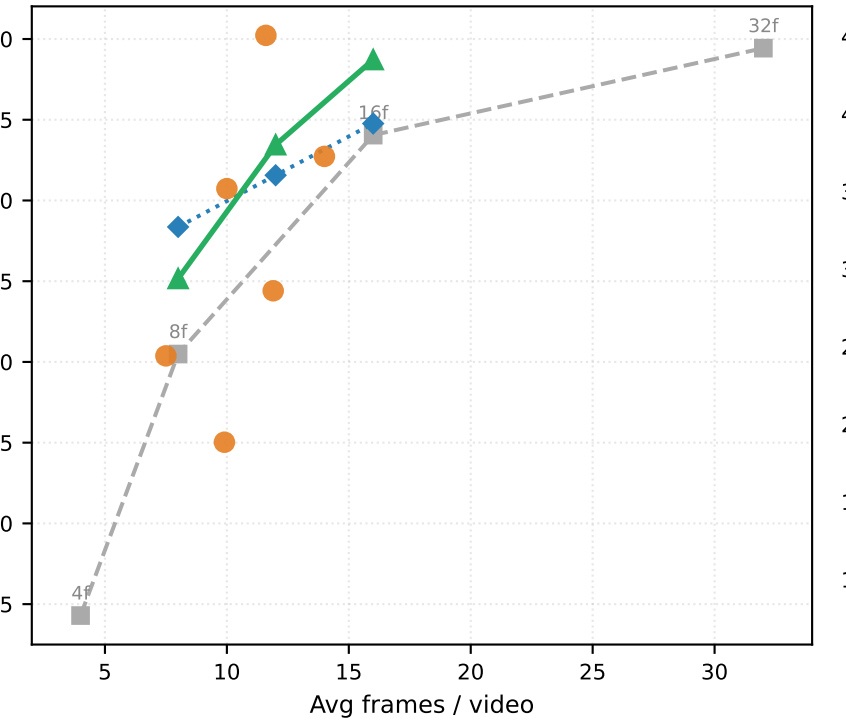
HMDB51
