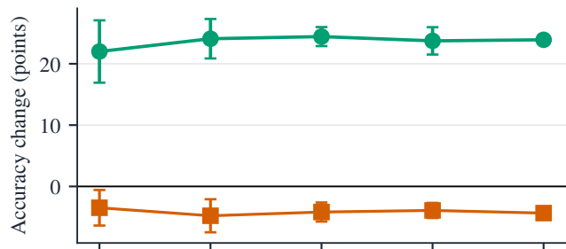
LLaVA-1.6-34B, QA
