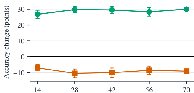
LLaVA-1.6-34B, QA
