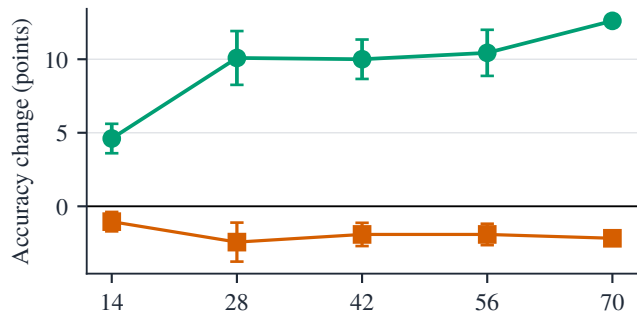
LLaVA-1.6-34B, MC
