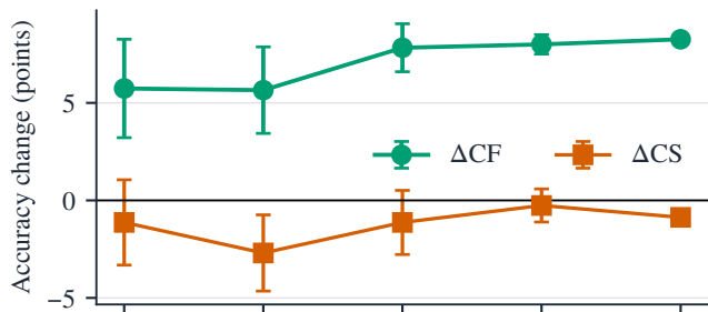
LLaVA-1.6-34B, MC
