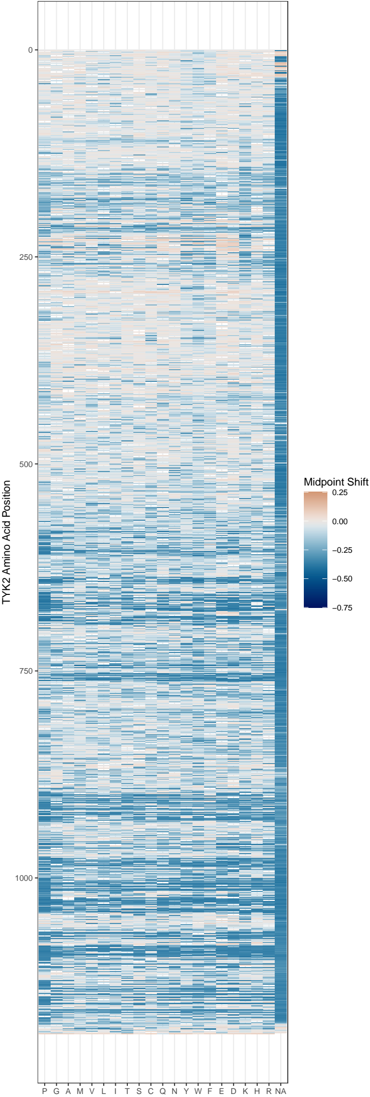
TYK2 // FlowDMS
