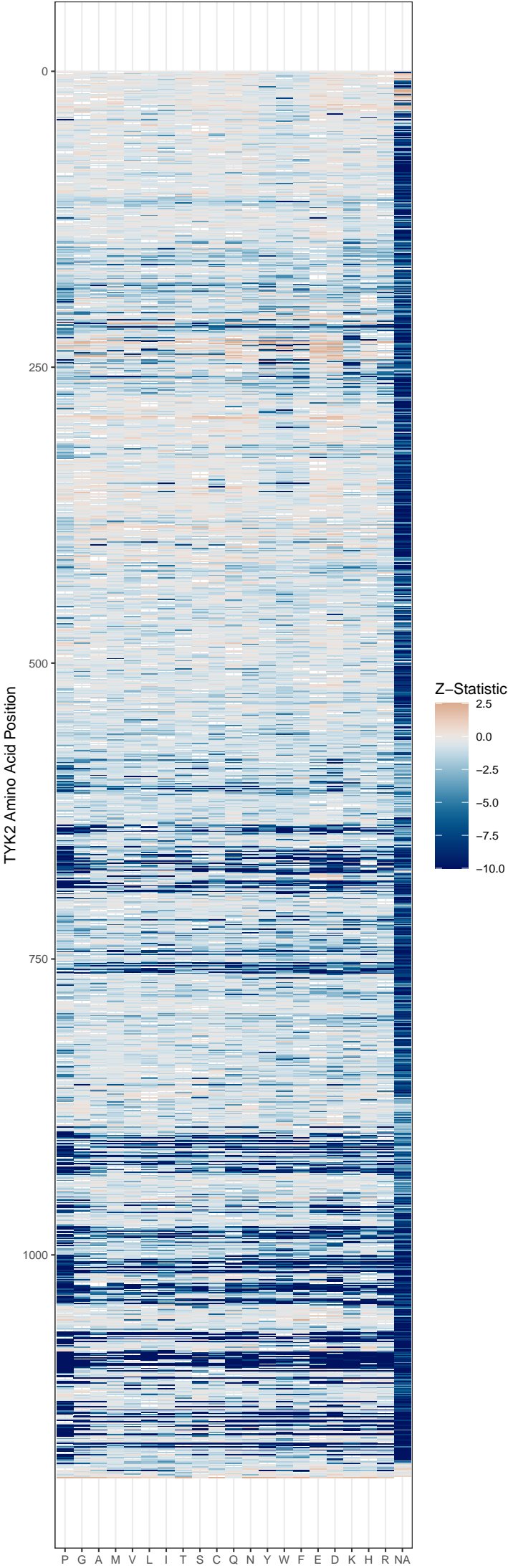
TYK2 // FlowDMS
