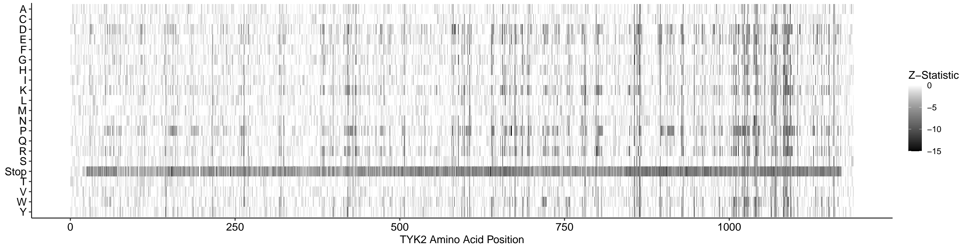
TYK2 // FlowDMS
