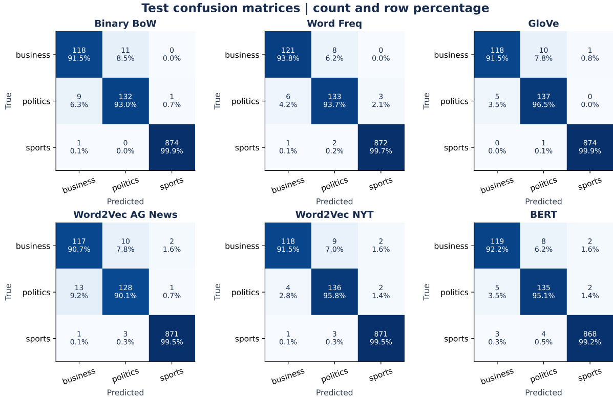
图 4: 六种方法的测试混淆矩阵。行为真实类别，列为预测类别；数字同时列出样本数及行归一化百分比。
