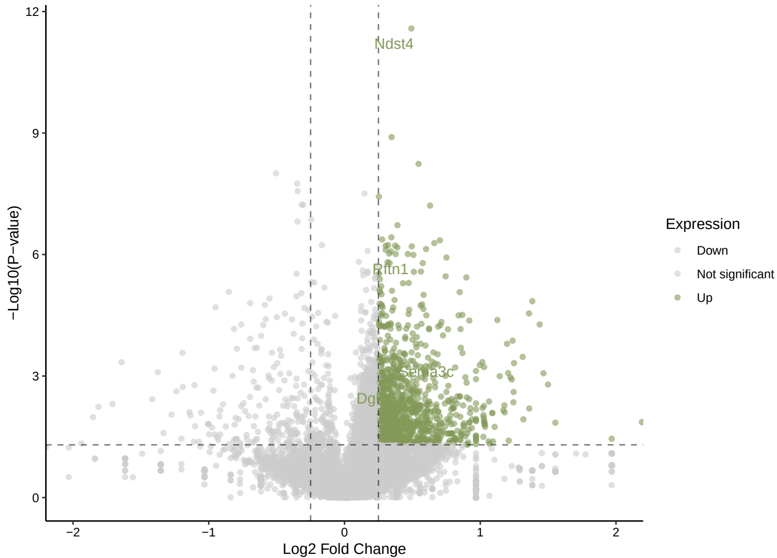
Volcano Plot: EGFP+ vs EGFP-
