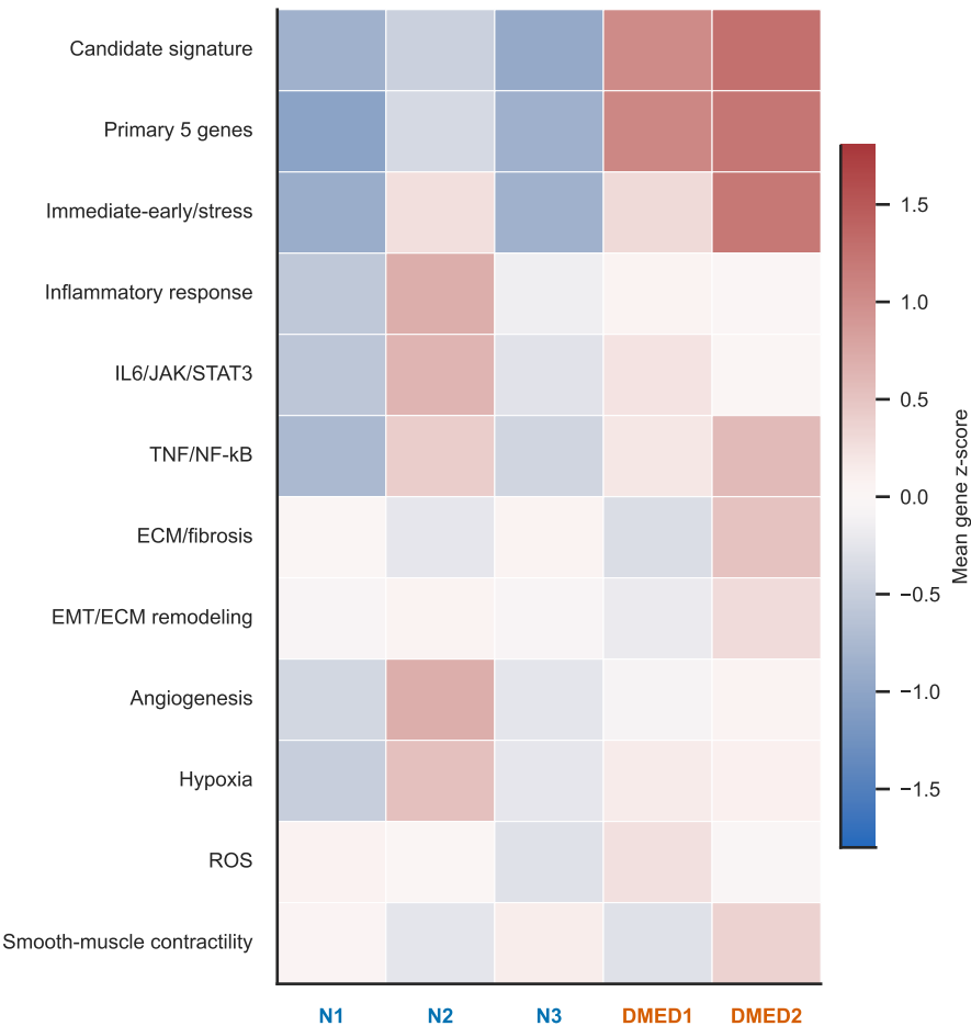
A. Donor module scores
