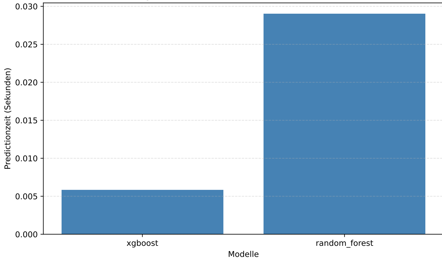
Vergleich der Modelle anhand der Predictionzeit
