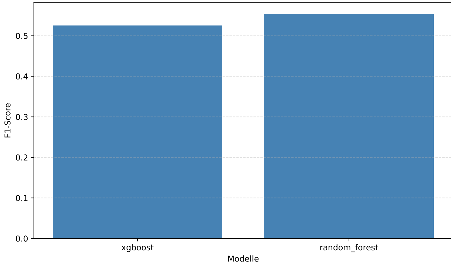
Vergleich der Modelle anhand des F1-Scores
