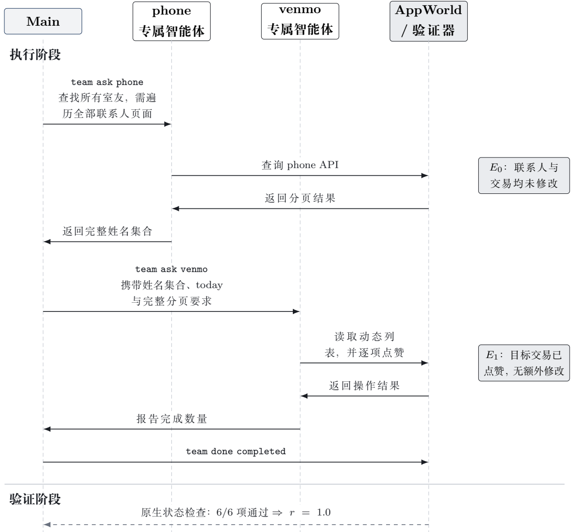
图 2: 参考轨迹中的信息流。上游角色取得事实，主智能体将其整理成下游可以执行的请求；奖励由终态 E_1 决定，不依赖轨迹文本。虚线表示任务结束后的验证阶段。
