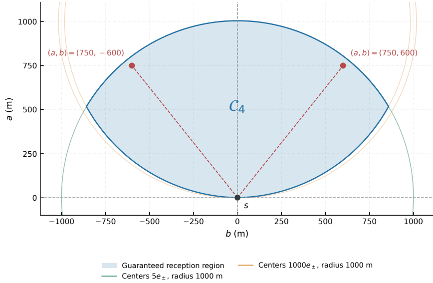
图4 首站局部坐标下的四圆保证接收区域，理论误差取 1^\circ ，标出一对可行示例点
