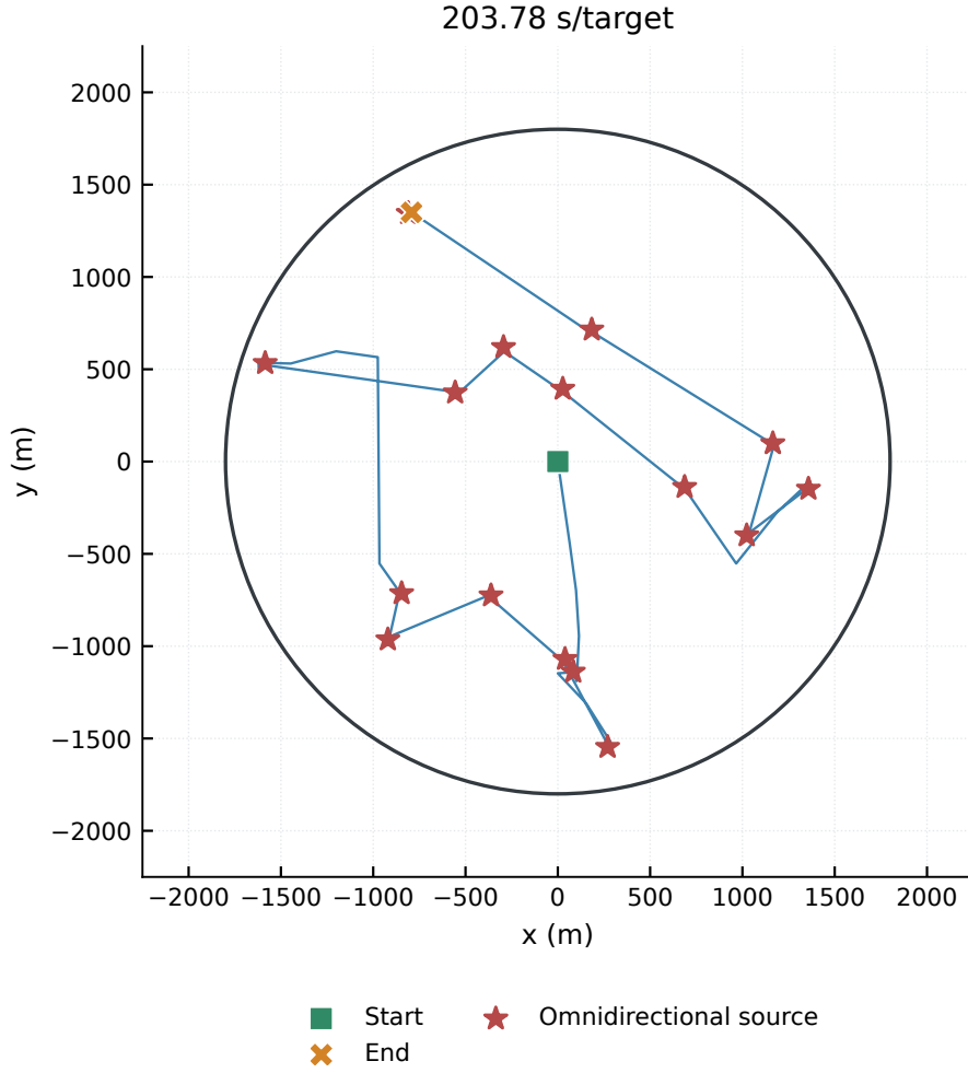
图 8 第三问代表性合成案例的实际动作轨迹；源位置由运行结束后的真值记录绘制
