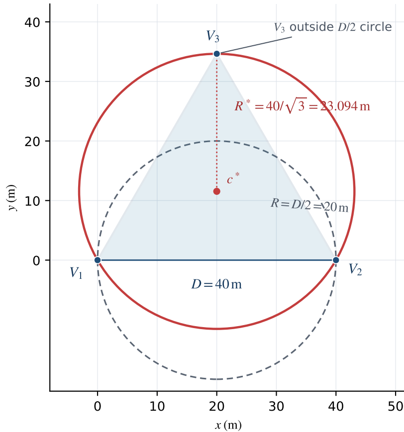
图 3 三次测向形成的等边三角形及其最小包围圆
