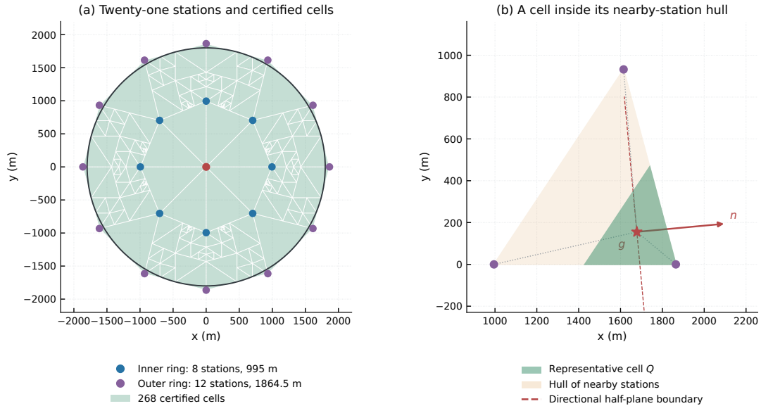
图 10 混合源的双环检测布局与近邻站凸包覆盖条件
