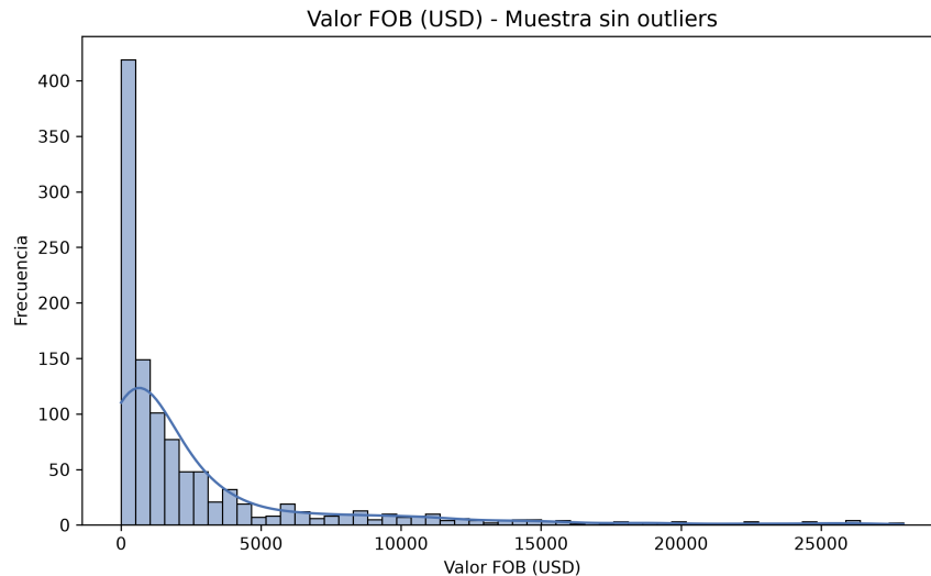
Figura 10: Distribución de Valor FOB (USD) – muestra sin outliers.
