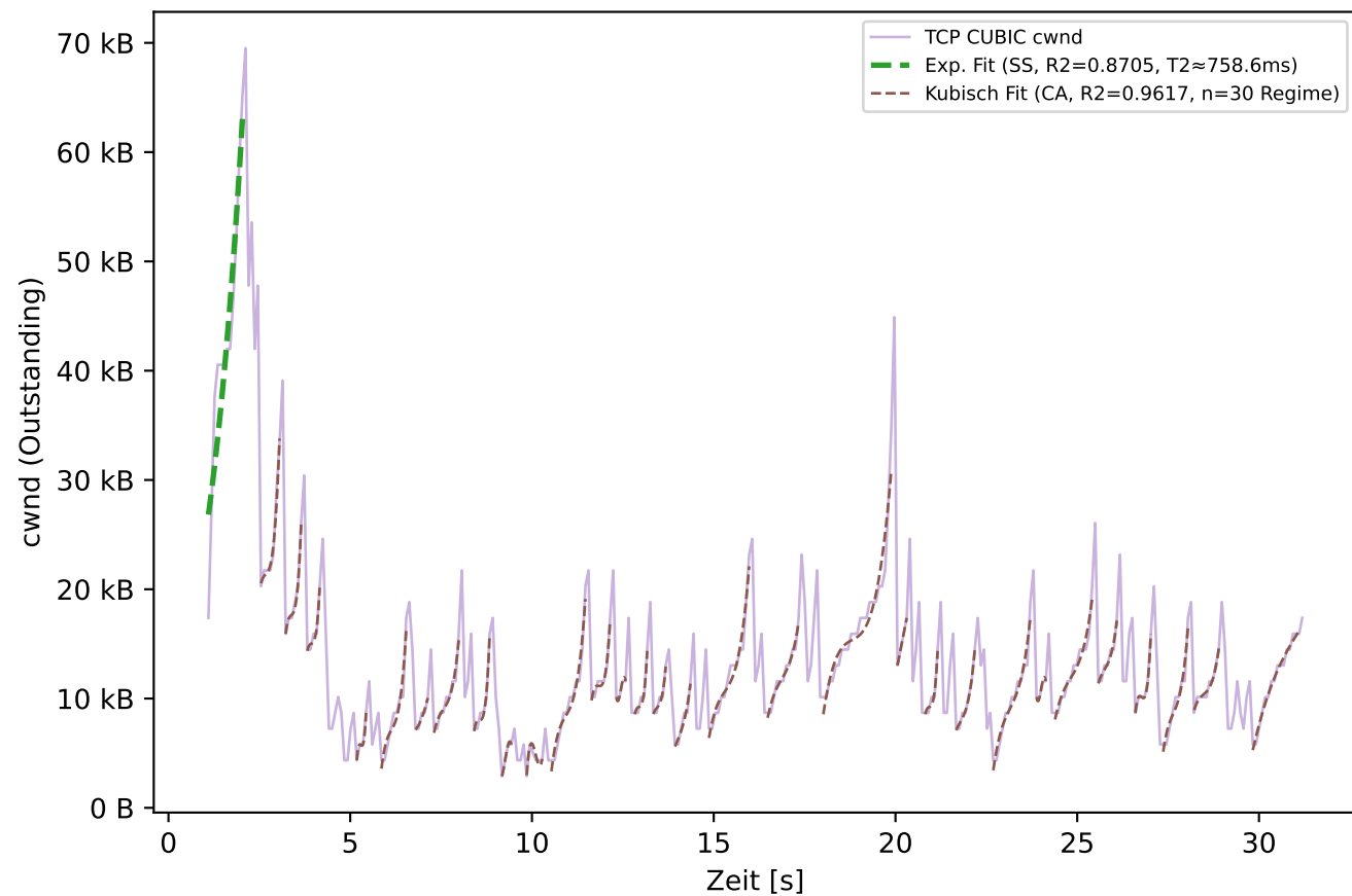
TCP CUBIC
