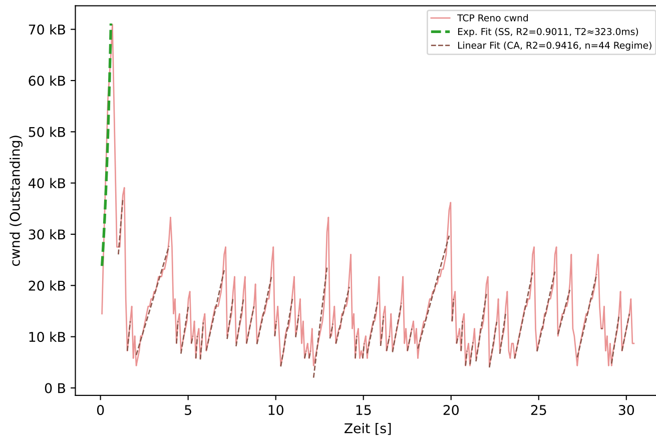
TCP Reno
