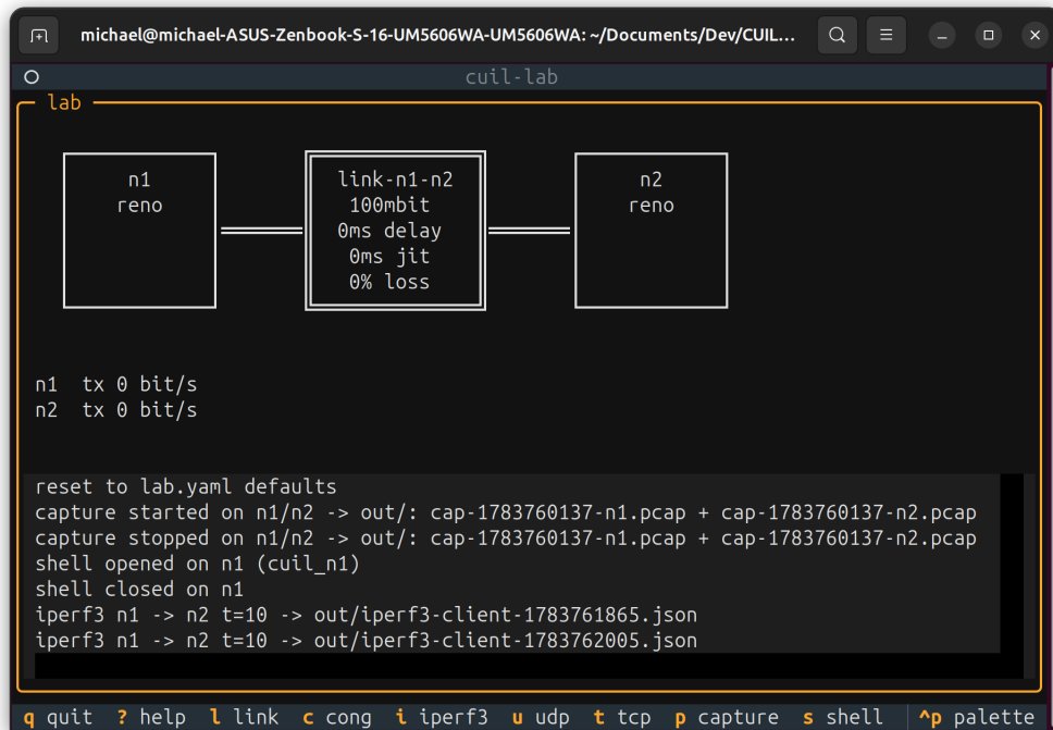
Abbildung 1: Docker Netzwerk
