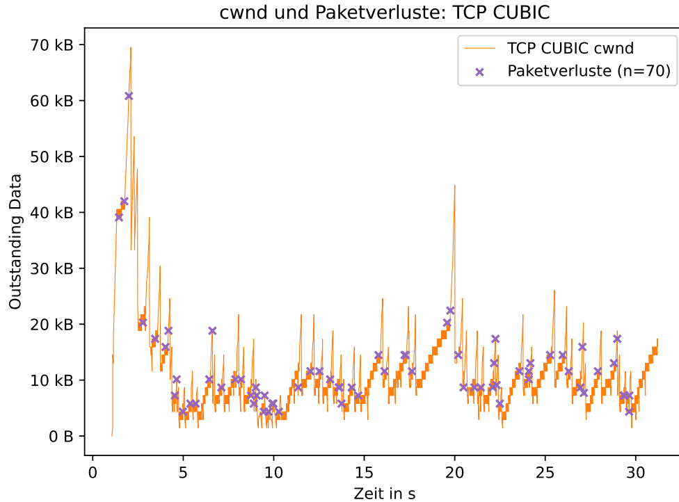
Abbildung 13: cwnd und Paketverluste von TCP CUBIC
