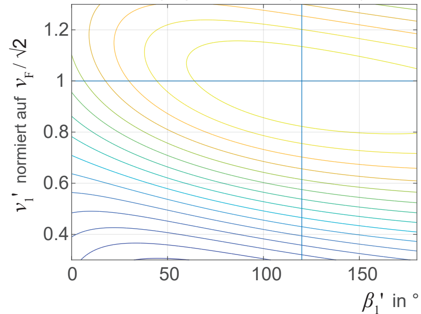
Energiegewinn \Delta H (normiert)
