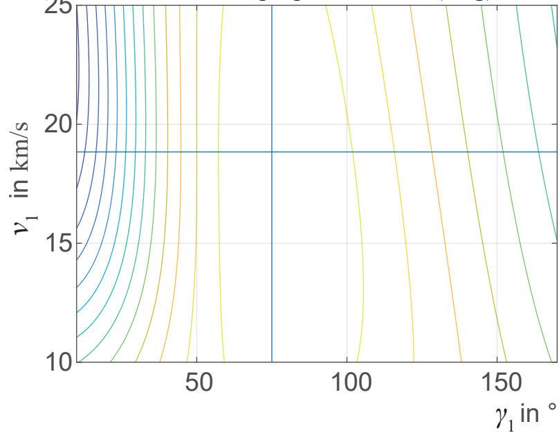
Energiegewinn \Delta H (J/kg)
