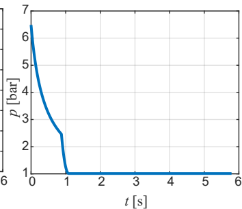
(c) Flaschendruck
