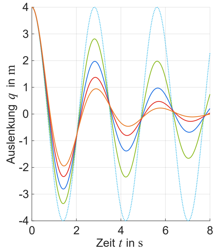
Stokes-Reibung
