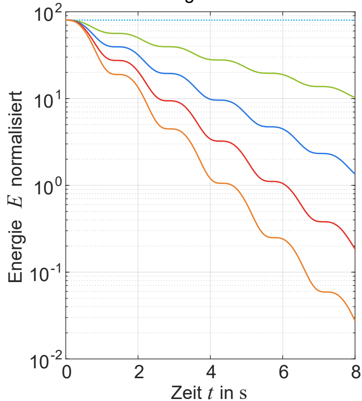
Stokes-Reibung
