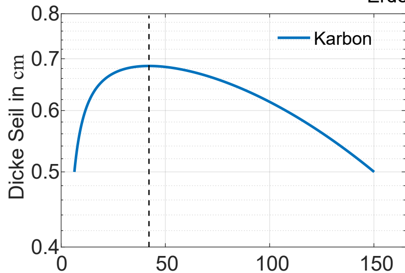
Erde
