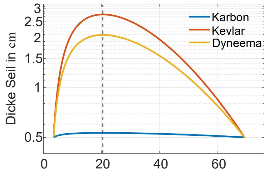
Mars
