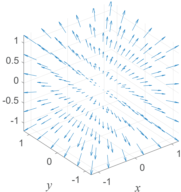
Vektorfunktion \mathbf{f} = (x, y, z)
