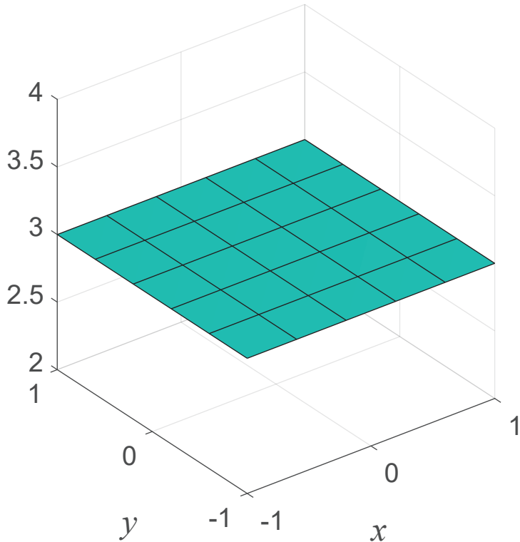
Divergenz \text{div } \mathbf{f} der Vektorfunktion
